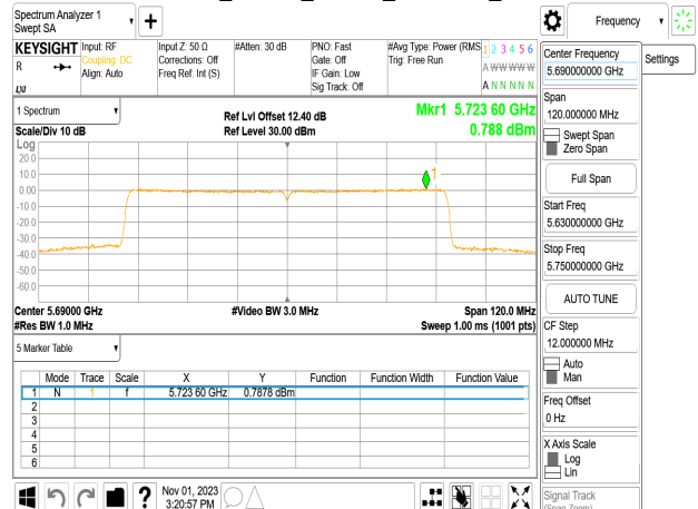
802.11ac_80MHz_Chain1_5690MHz_UNII 2C
