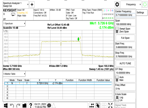
802.11n_40MHz_Chain1_5710MHz_UNII 3
