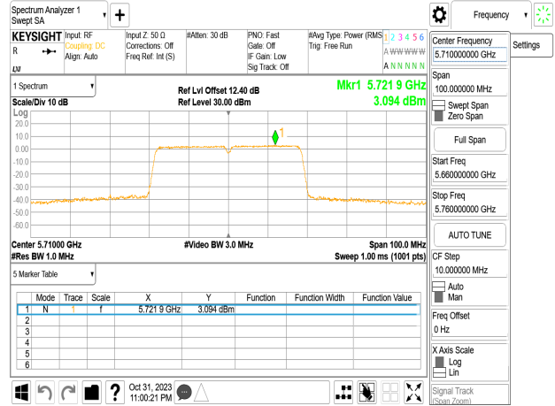
802.11n_40MHz_Chain1_5710MHz_UNII 3
