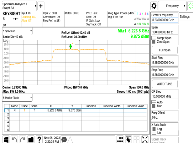
802.11n_40MHz_Chain3_5230MHz
