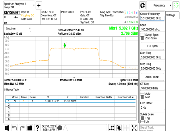
802.11n_40MHz_Chain2_5310MHz
