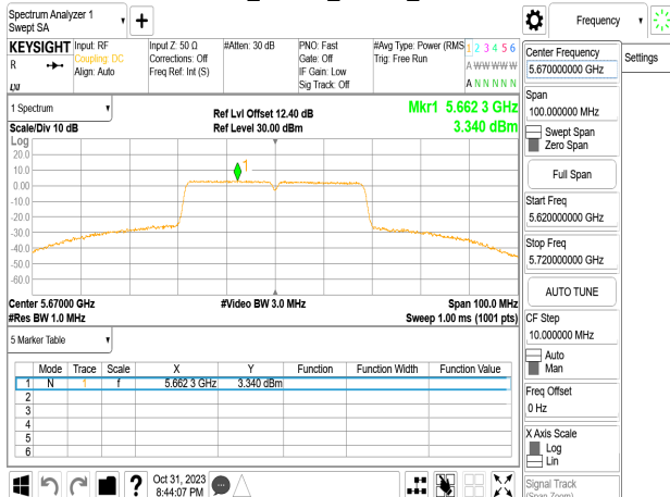
802.11n_40MHz_Chain2_5670MHz
