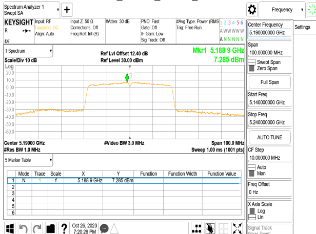
802.11n_40MHz_Chain2_5190MHz
