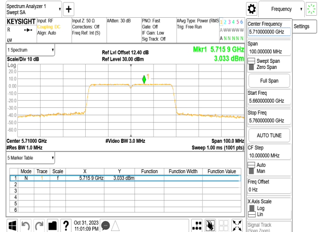
802.11n_40MHz_Chain2_5710MHz_UNII 3
