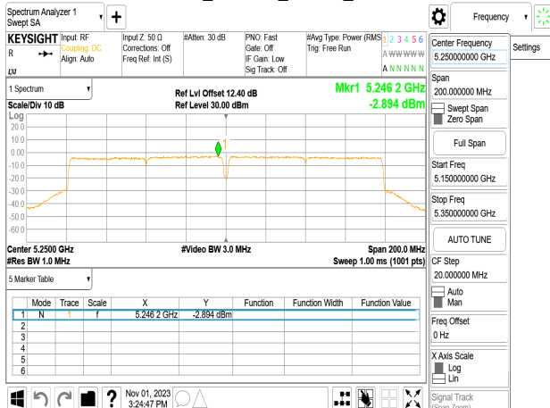
802.11ac_160MHz_Chain2_5250MHz
