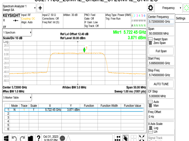
802.11be_20MHz_Chain2_5720MHz_UNII 3
