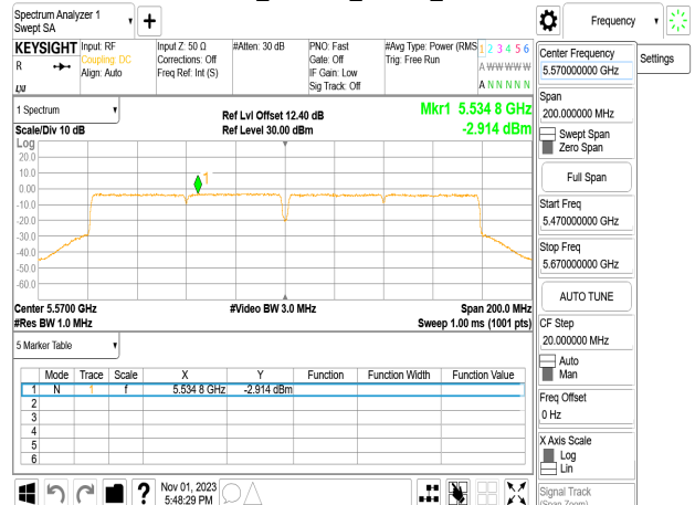
802.11ac_160MHz_Chain3_5570MHz
