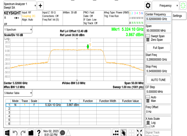
802.11be_20MHz_Chain3_5320MHz
