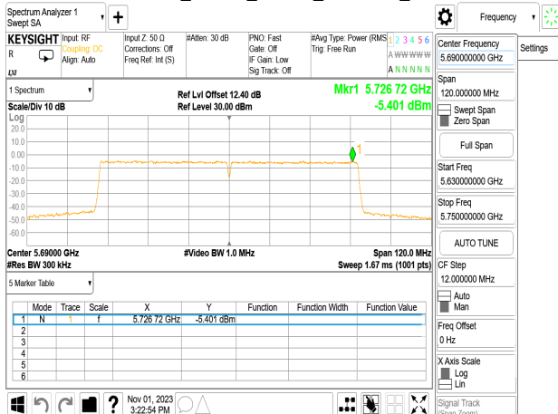
802.11ac_80MHz_Chain3_5690MHz_UNII 3
