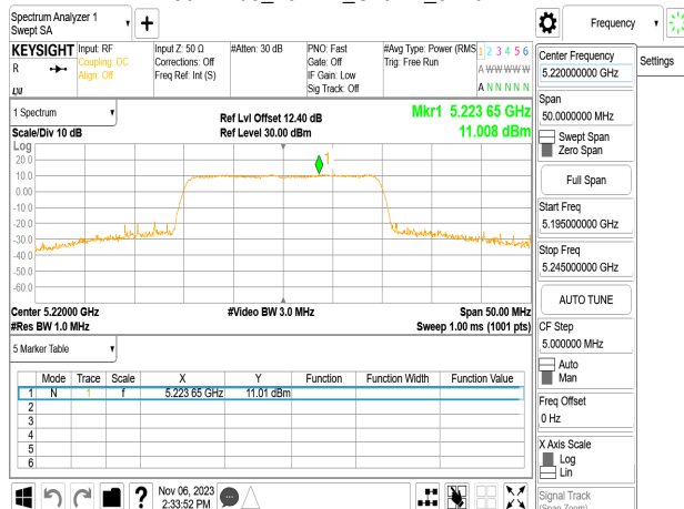
802.11be_20MHz_Chain2_5220MHz
