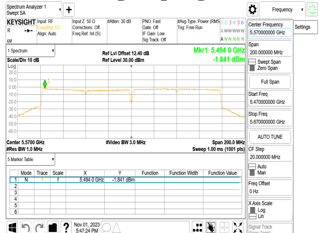
802.11ac_160MHz_Chain0_5570MHz
