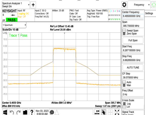
802.11ac_80MHz_Chain1_6465MHz
