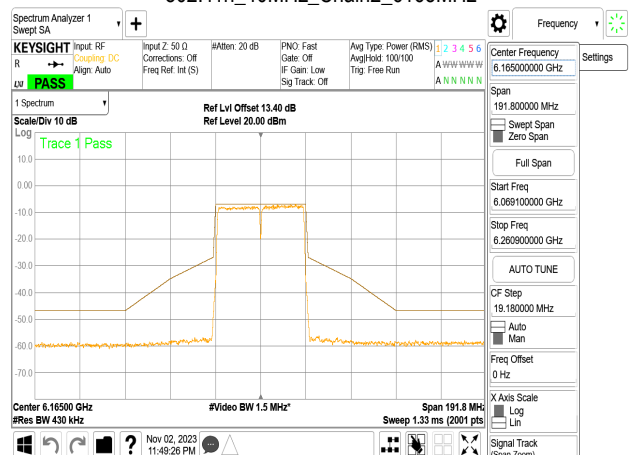
802.11n_40MHz_Chain2_6165MHz
