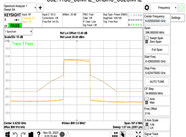
802.11ac_80MHz_Chain0_6625MHz
