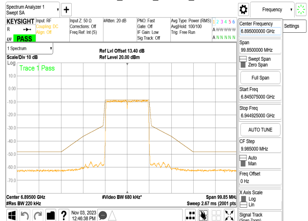
802.11be_20MHz_Chain1_6895MHz
