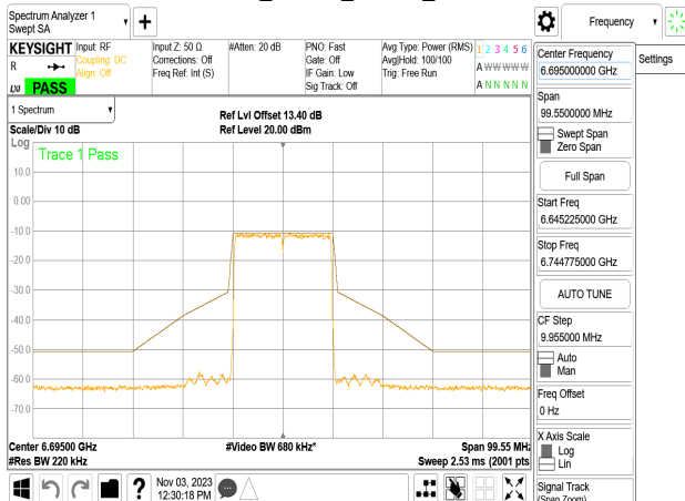
802.11be_20MHz_Chain1_6695MHz
