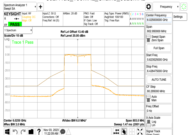
802.11ac_160MHz_Chain3_6025MHz
