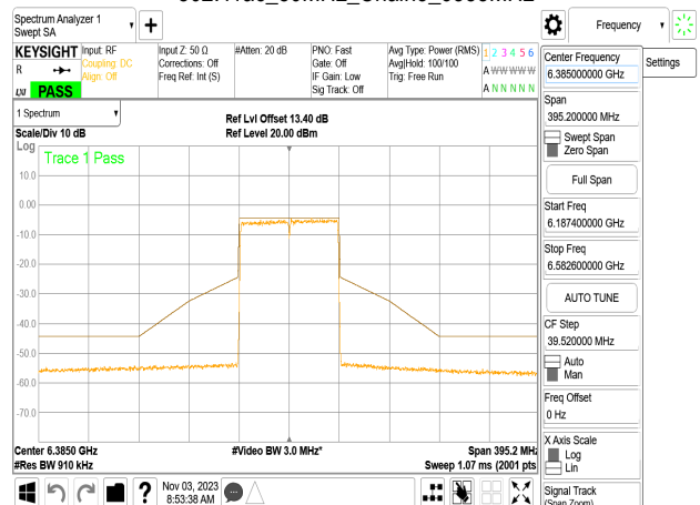
802.11ac_80MHz_Chain3_6385MHz
