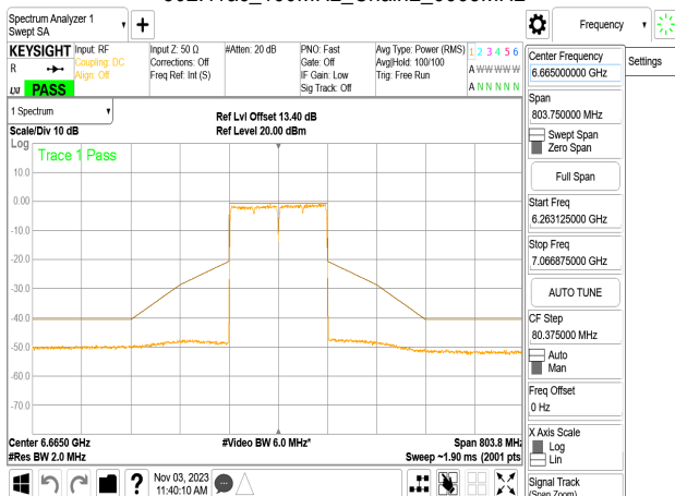
802.11ac_160MHz_Chain2_6665MHz
