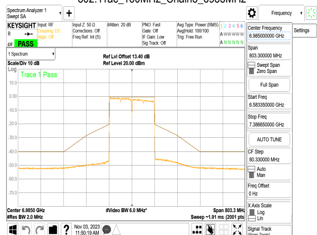
802.11ac_160MHz_Chain3_6985MHz
