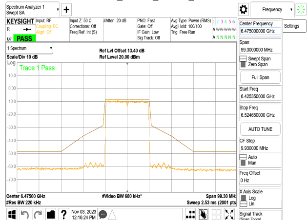
802.11be_20MHz_Chain1_6475MHz
