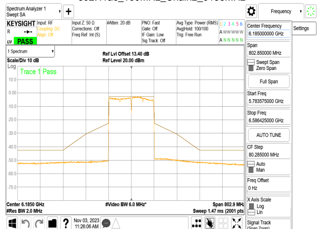
802.11ac_160MHz_Chain2_6185MHz
