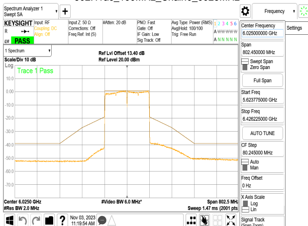
802.11ac_160MHz_Chain0_6025MHz
