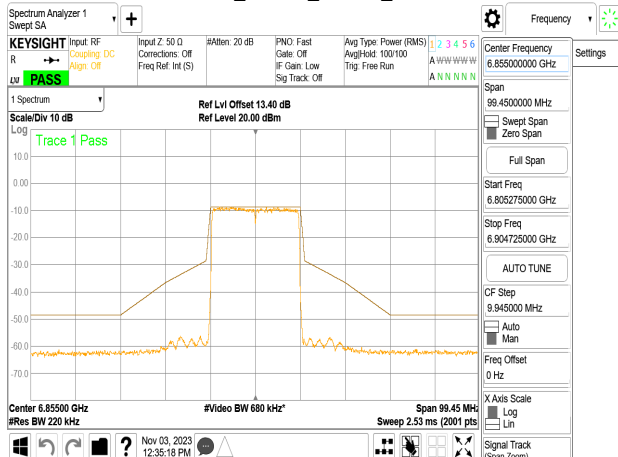
802.11be_20MHz_Chain0_6855MHz
