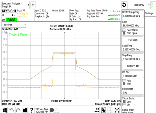
802.11be_20MHz_Chain1_6175MHz
