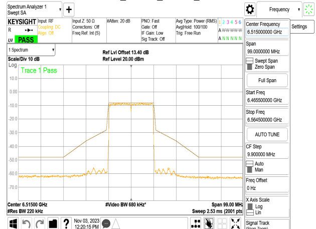
802.11be_20MHz_Chain0_6515MHz
