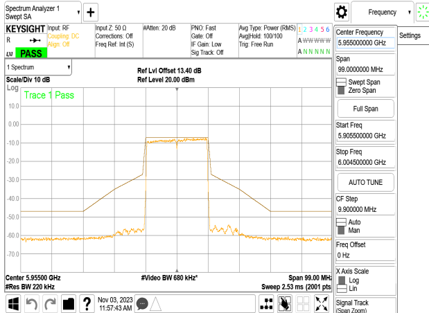
802.11be_20MHz_Chain2_5955MHz
