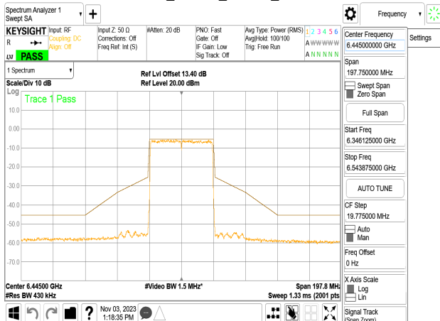
802.11be_40MHz_Chain1_6445MHz
