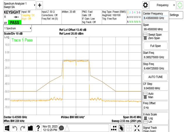
802.11be_20MHz_Chain2_6435MHz
