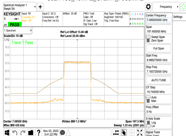
802.11be_40MHz_Chain1_7085MHz
