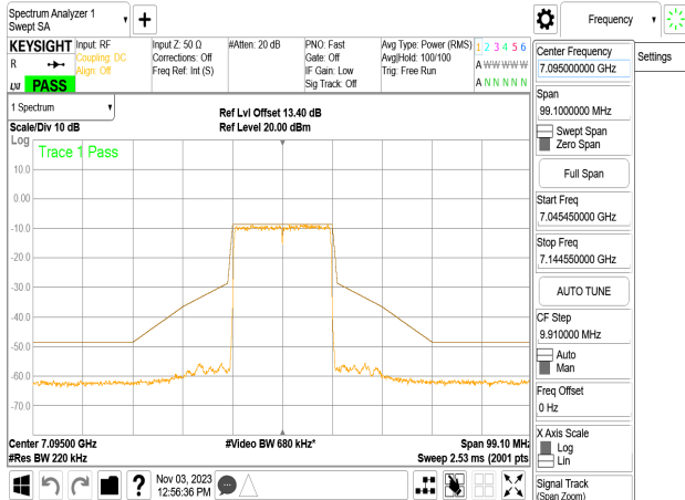
802.11be_20MHz_Chain2_7095MHz
