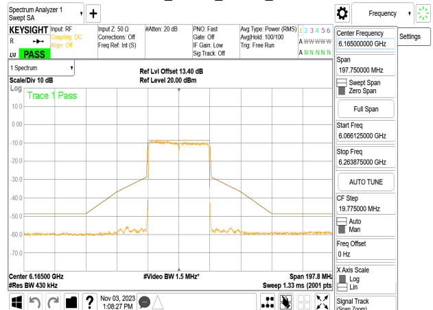
802.11be_40MHz_Chain0_6165MHz
