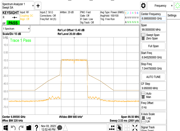
802.11be_20MHz_Chain3_6995MHz
