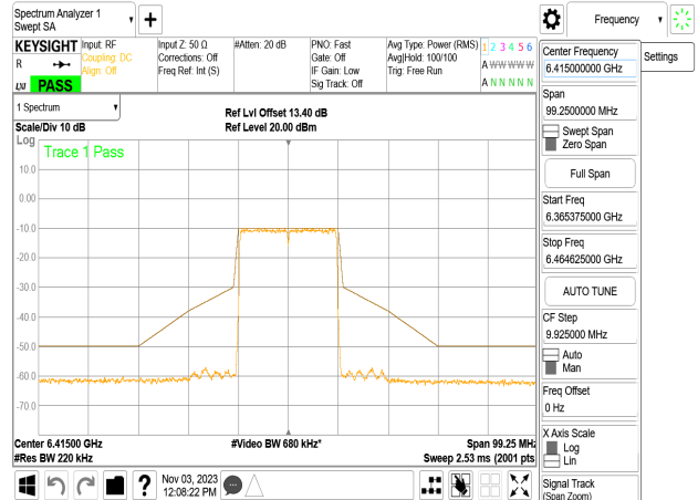
802.11be_20MHz_Chain3_6415MHz
