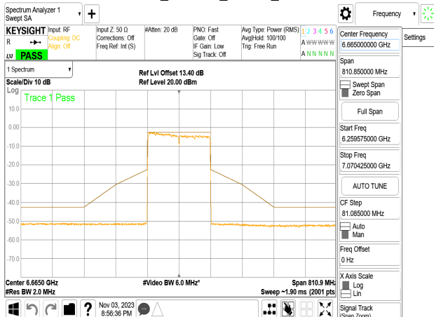
802.11be_160MHz_Chain0_6665MHz
