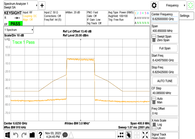
802.11be_80MHz_Chain2_6625MHz
