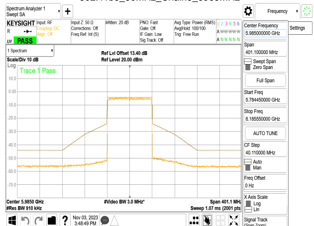
802.11be_80MHz_Chain3_5985MHz
