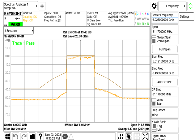
802.11be_160MHz_Chain1_6025MHz
