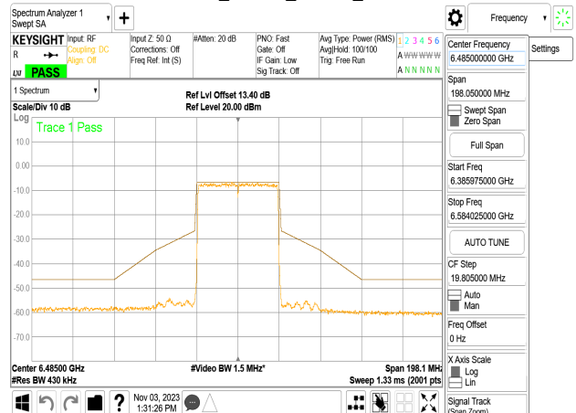
802.11be_40MHz_Chain3_6485MHz
