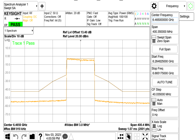
802.11be_80MHz_Chain0_6465MHz
