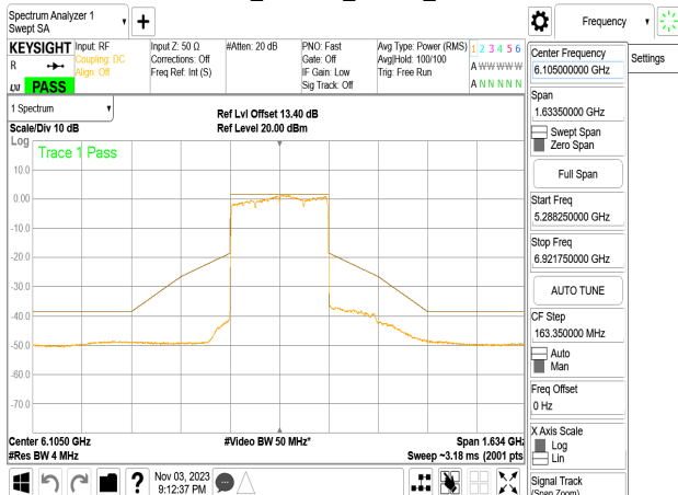
802.11be_320MHz_Chain0_6105MHz
