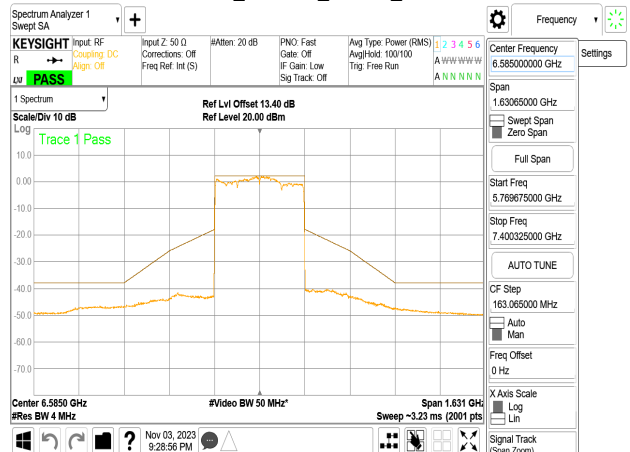
802.11be_320MHz_Chain0_6585MHz
