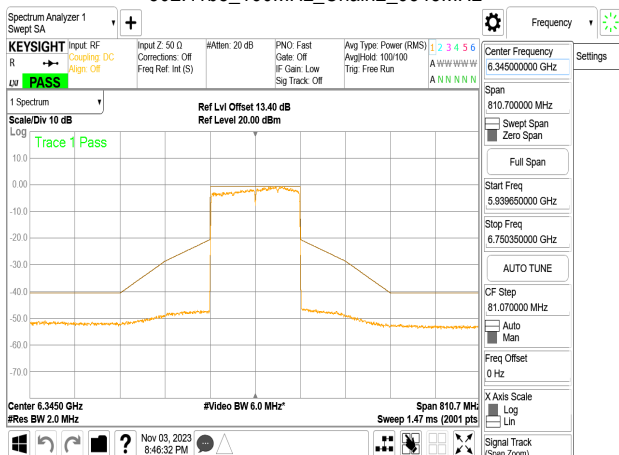
802.11be_160MHz_Chain2_6345MHz
