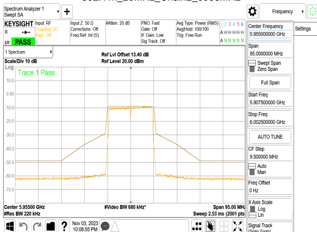
802.11n_20MHz_Chain2_5955MHz
