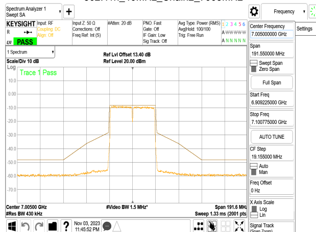
802.11n_40MHz_Chain2_7005MHz
