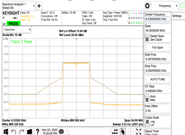
802.11n_20MHz_Chain2_6535MHz
