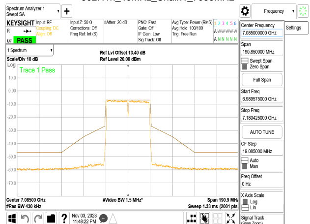
802.11n_40MHz_Chain1_7085MHz
