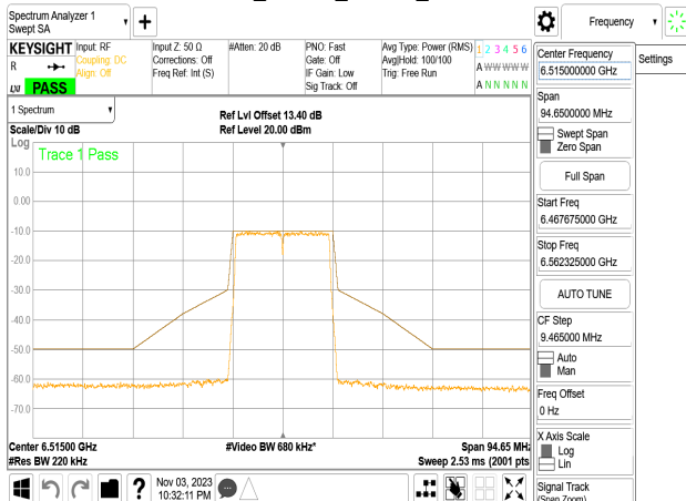
802.11n_20MHz_Chain3_6515MHz
