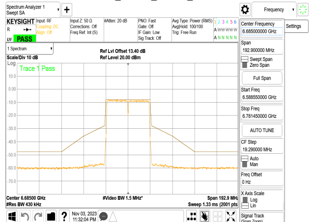
802.11n_40MHz_Chain0_6685MHz
