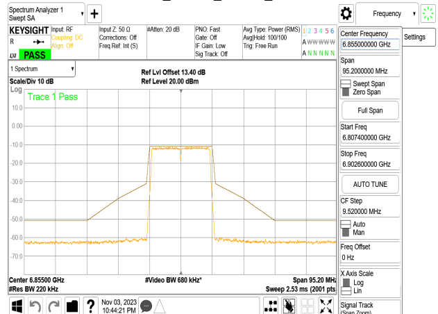
802.11n_20MHz_Chain3_6855MHz
