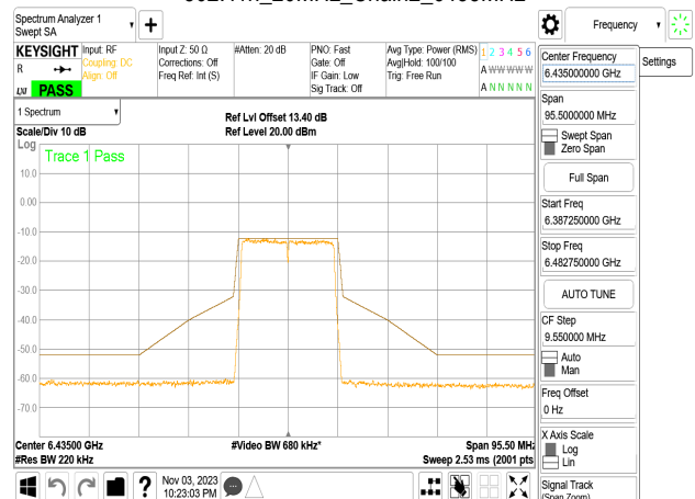
802.11n_20MHz_Chain2_6435MHz
