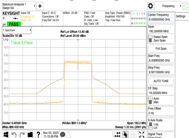
802.11n_40MHz_Chain2_6405MHz
