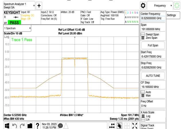
802.11n_40MHz_Chain2_6525MHz
