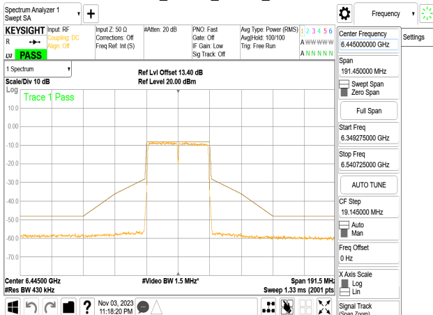
802.11n_40MHz_Chain1_6445MHz
