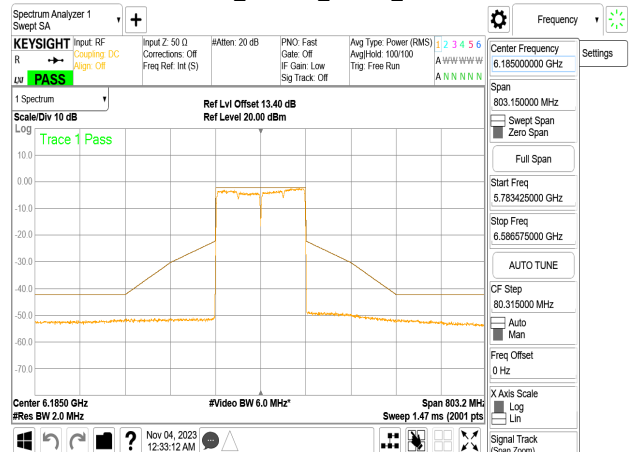
802.11ac_160MHz_Chain0_6185MHz
