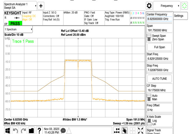
802.11n_40MHz_Chain3_6925MHz
