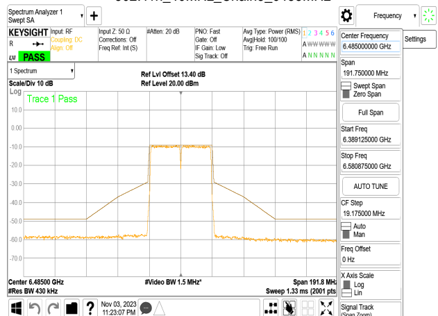
802.11n_40MHz_Chain3_6485MHz
