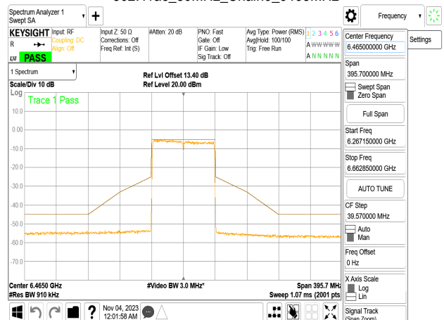
802.11ac_80MHz_Chain0_6465MHz
