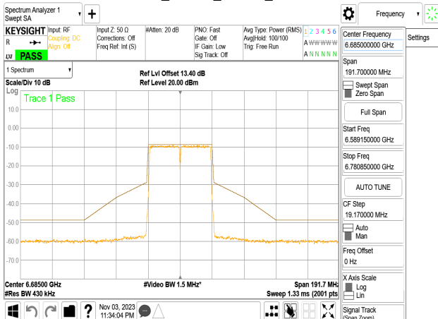
802.11n_40MHz_Chain3_6685MHz
