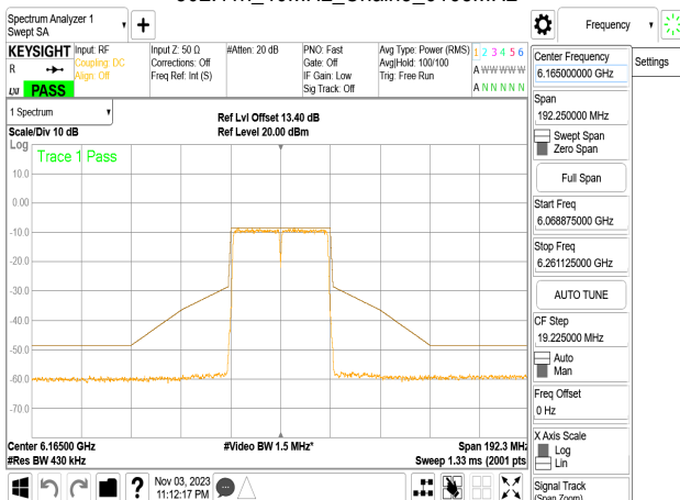
802.11n_40MHz_Chain3_6165MHz
