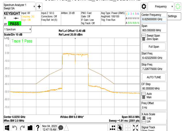
802.11ac_160MHz_Chain2_6825MHz
