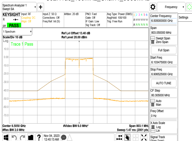
802.11ac_160MHz_Chain1_6505MHz
