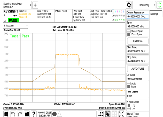
802.11be_20MHz_Chain0_6435MHz
