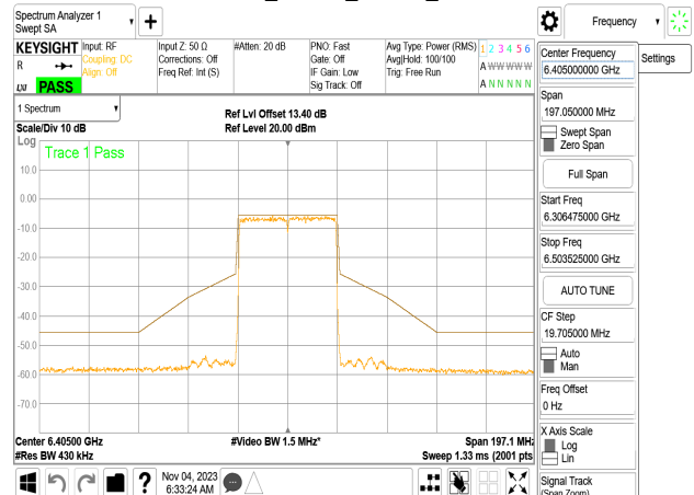
802.11be_40MHz_Chain3_6405MHz
