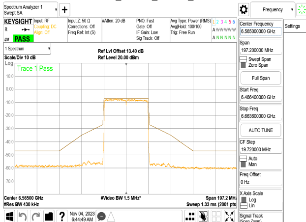
802.11be_40MHz_Chain2_6565MHz
