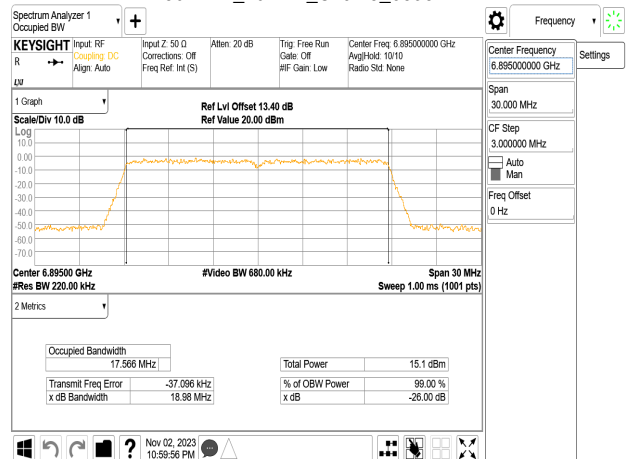
802.11n_20MHz_Chain3_6895MHz
