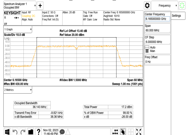
802.11n_40MHz_Chain2_6165MHz
