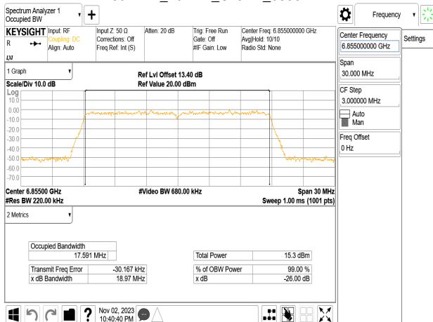
802.11n_20MHz_Chain2_6855MHz
