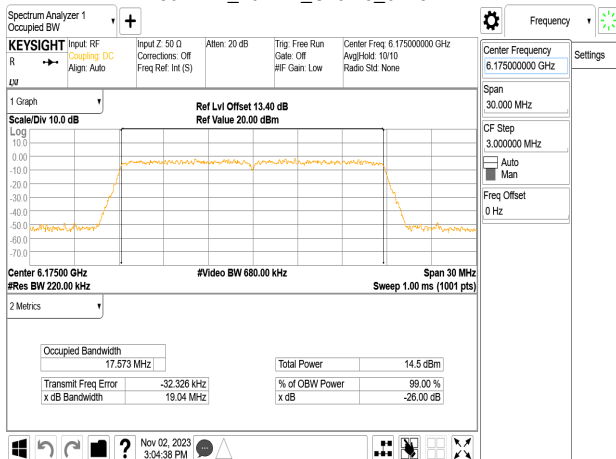
802.11n_20MHz_Chain3_6175MHz
