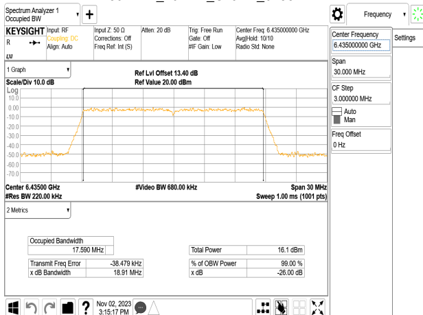
802.11n_20MHz_Chain1_6435MHz
