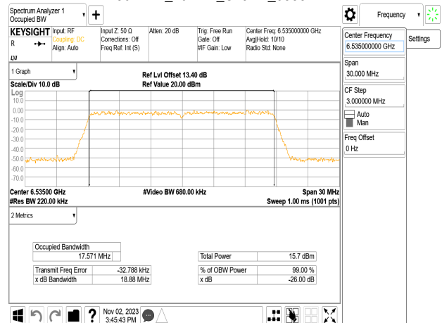
802.11n_20MHz_Chain1_6535MHz
