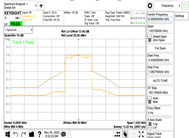
802.11be_320MHz_Chain0_6265MHz
