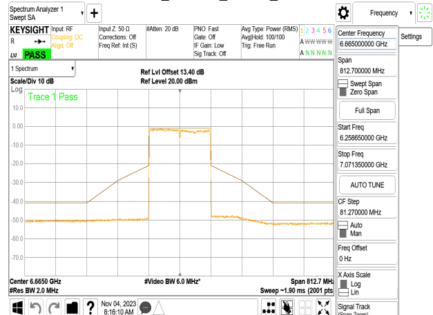
802.11be_160MHz_Chain1_6665MHz
