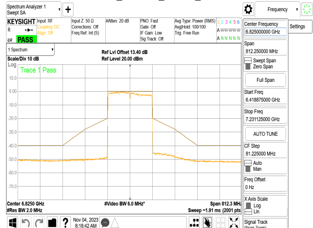
802.11be_160MHz_Chain0_6825MHz
