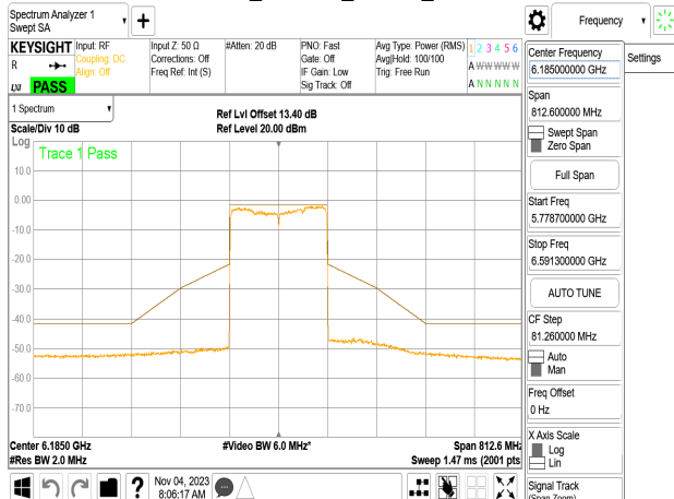
802.11be_160MHz_Chain1_6185MHz
