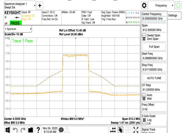
802.11be_160MHz_Chain2_6505MHz
