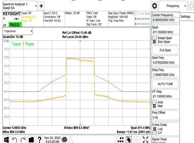
802.11be_160MHz_Chain2_6985MHz
