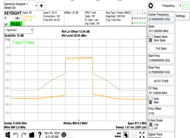
802.11be_160MHz_Chain3_6345MHz
