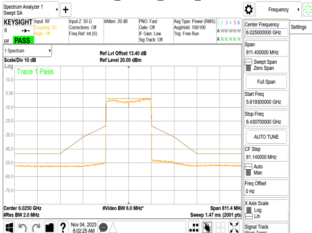
802.11be_160MHz_Chain2_6025MHz
