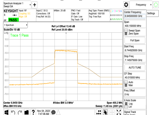
802.11be_80MHz_Chain2_6945MHz
