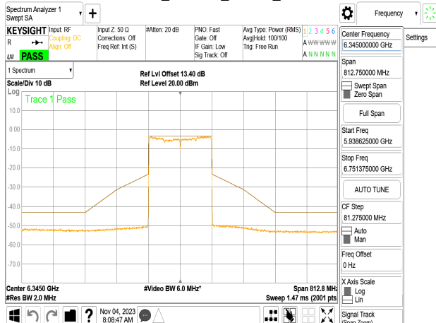
802.11be_160MHz_Chain0_6345MHz
