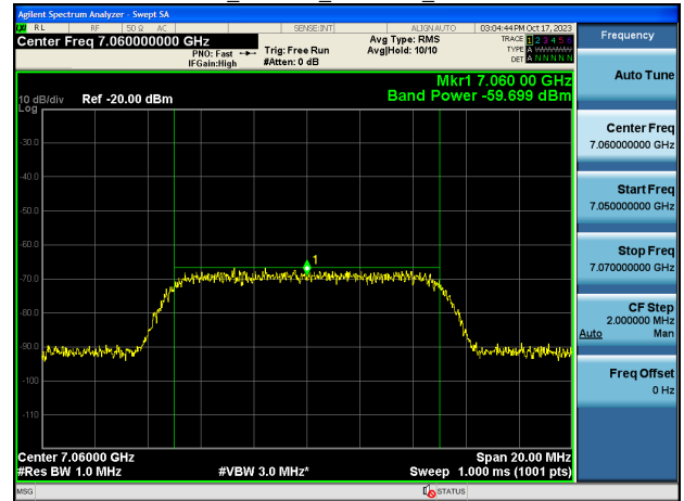
802.11be_320MHz_6905MHz_AWGN:7060
