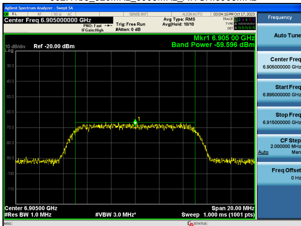
802.11be_320MHz_6905MHz_AWGN:6905MHz
