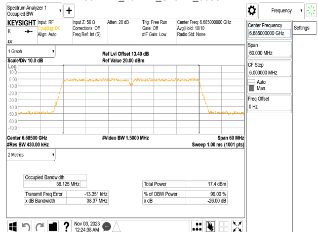
802.11n_40MHz_Chain2_6685MHz
