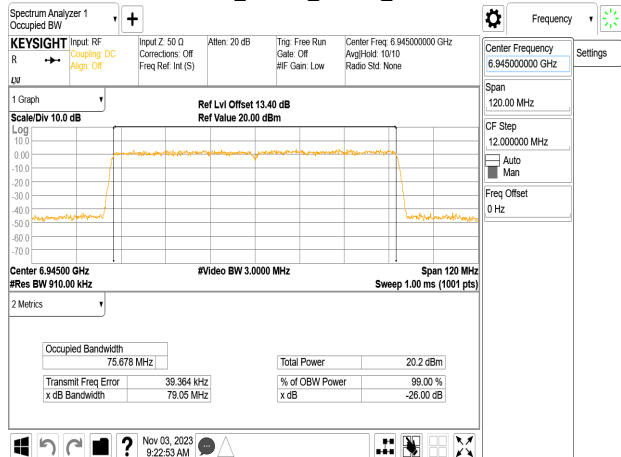
802.11ac_80MHz_Chain1_6945MHz
