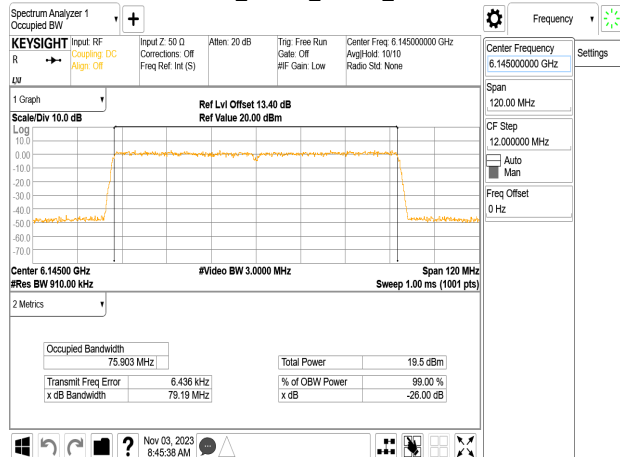
802.11ac_80MHz_Chain2_6145MHz
