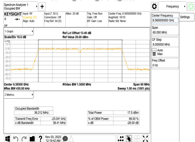
802.11n_40MHz_Chain3_6565MHz
