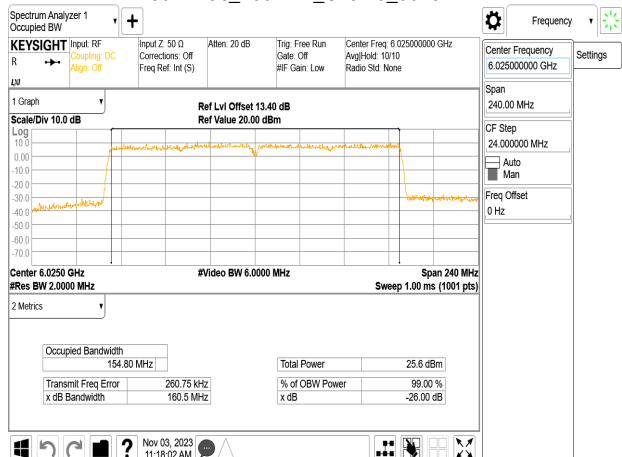
802.11ac_160MHz_Chain0_6025MHz
