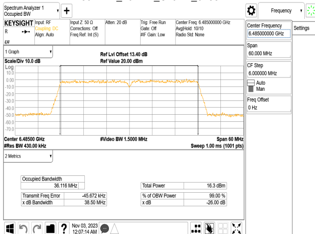
802.11n_40MHz_Chain2_6485MHz
