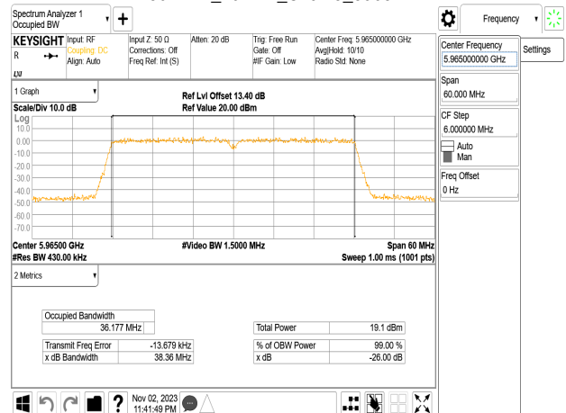
802.11n_40MHz_Chain3_5965MHz
