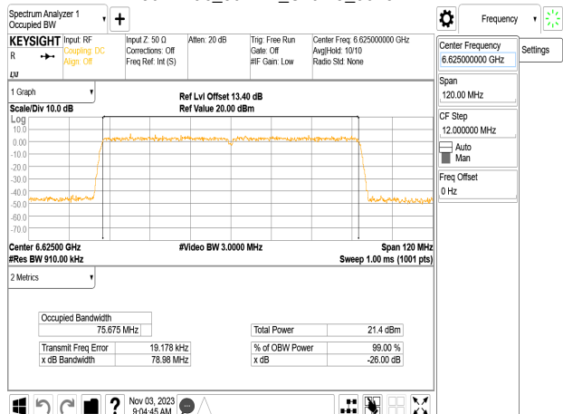
802.11ac_80MHz_Chain3_6625MHz
