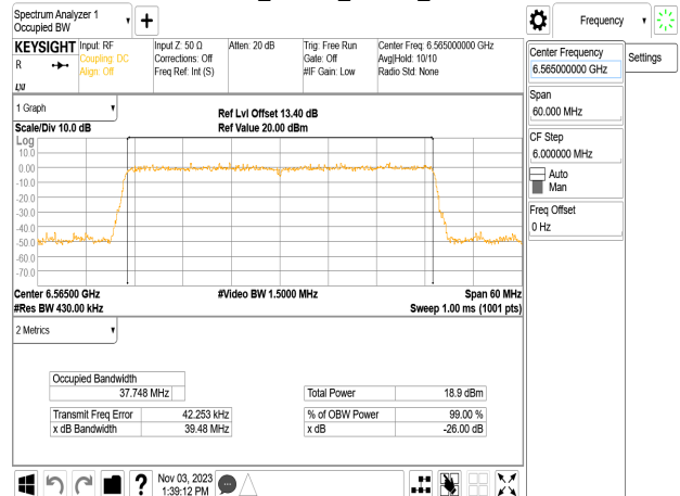
802.11be_40MHz_Chain1_6565MHz
