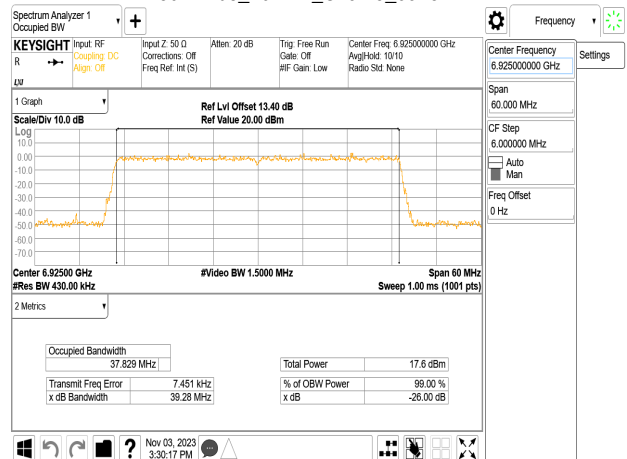
802.11be_40MHz_Chain3_6925MHz
