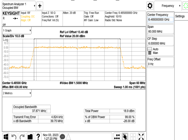
802.11be_40MHz_Chain0_6485MHz
