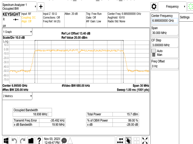
802.11be_20MHz_Chain3_6995MHz
