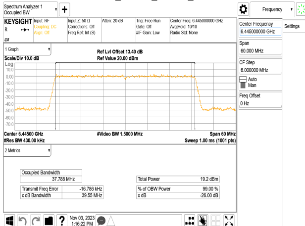
802.11be_40MHz_Chain1_6445MHz
