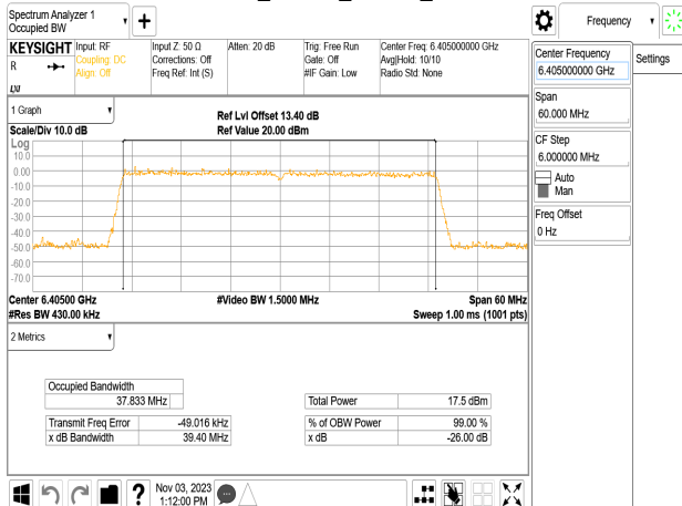
802.11be_40MHz_Chain2_6405MHz
