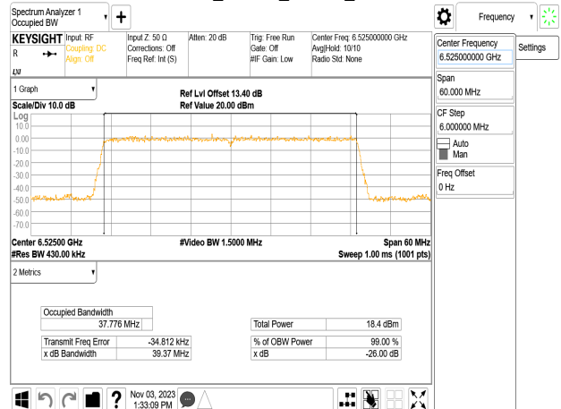
802.11be_40MHz_Chain2_6525MHz
