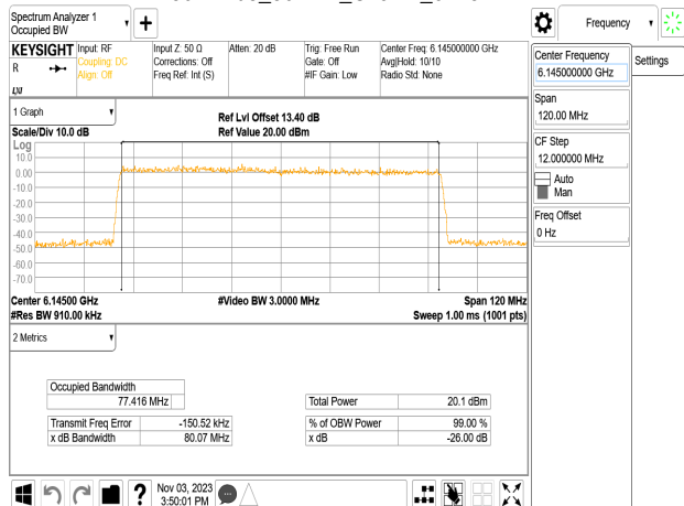
802.11be_80MHz_Chain1_6145MHz
