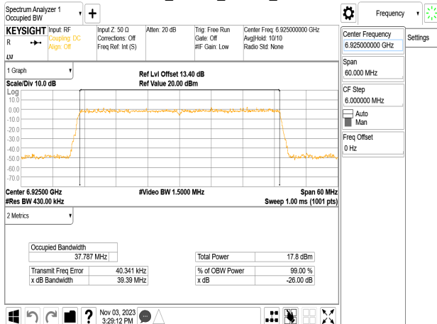
802.11be_40MHz_Chain0_6925MHz
