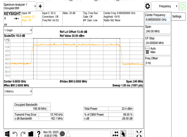
802.11be_160MHz_Chain3_6665MHz
