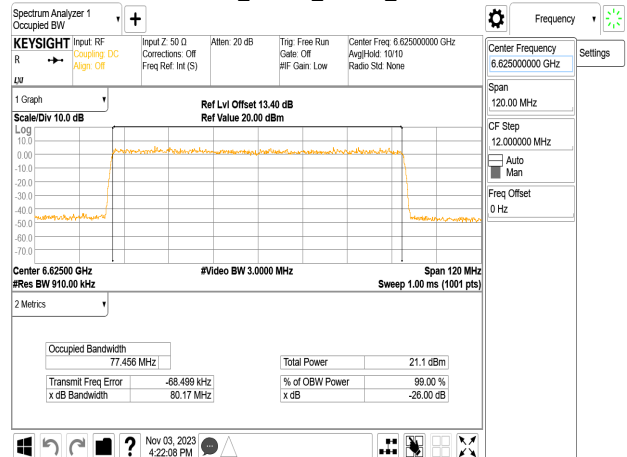
802.11be_80MHz_Chain2_6625MHz
