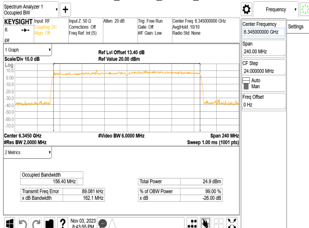
802.11be_160MHz_Chain2_6345MHz
