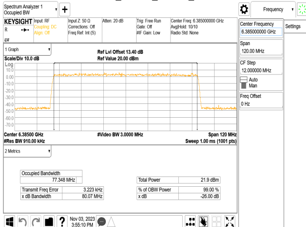
802.11be_80MHz_Chain2_6385MHz
