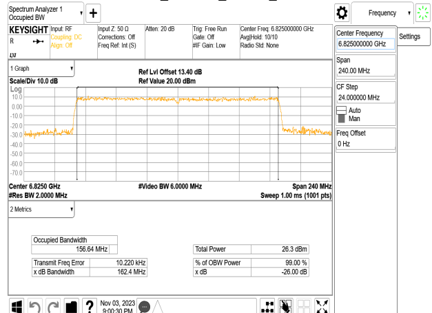
802.11be_160MHz_Chain2_6825MHz
