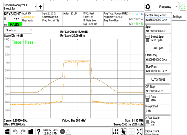
802.11a_20MHz_Chain3_6855MHz
