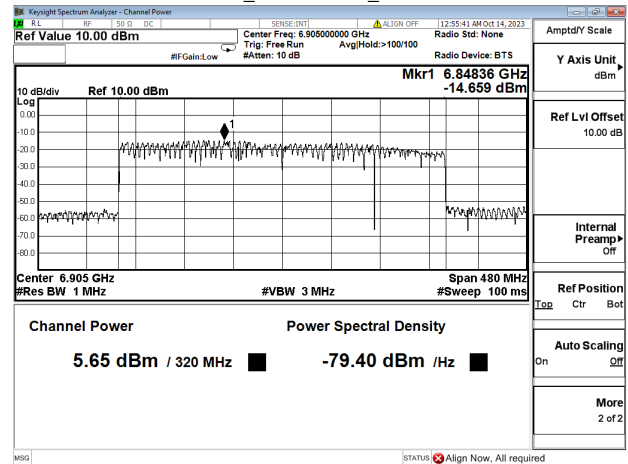
Channel Power+PSD_802.11be320_802.11be320 6905MHz
