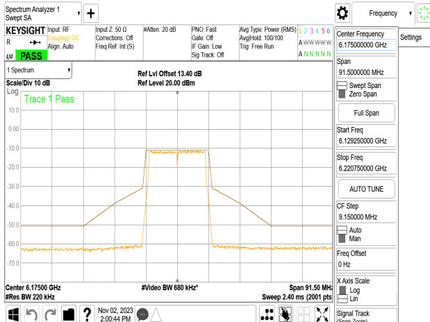
802.11a_20MHz_Chain1_6175MHz
