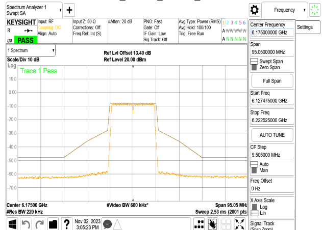
802.11n_20MHz_Chain0_6175MHz
