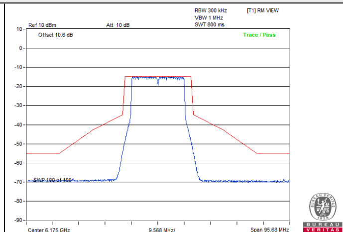
802.11be (EHT20) / Chain 2 : CH 45
