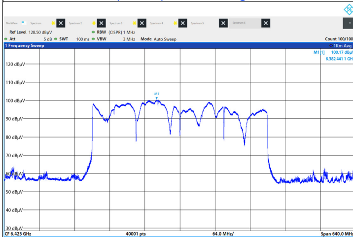
802.11be (EHT320) Beamforming : CH 95
