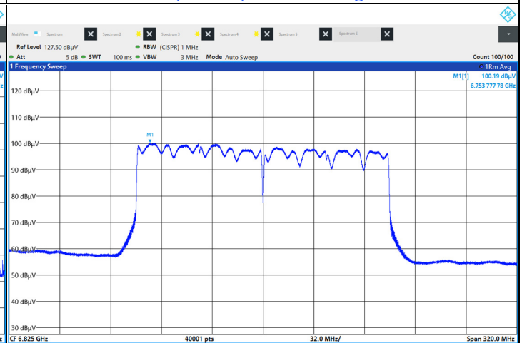
802.11be (EHT160) Beamforming : CH 175
