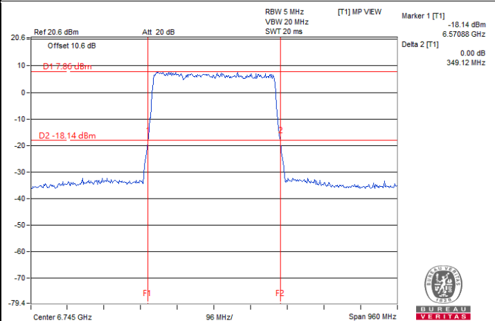
802.11be (EHT320) / Chain 3 : CH 159
