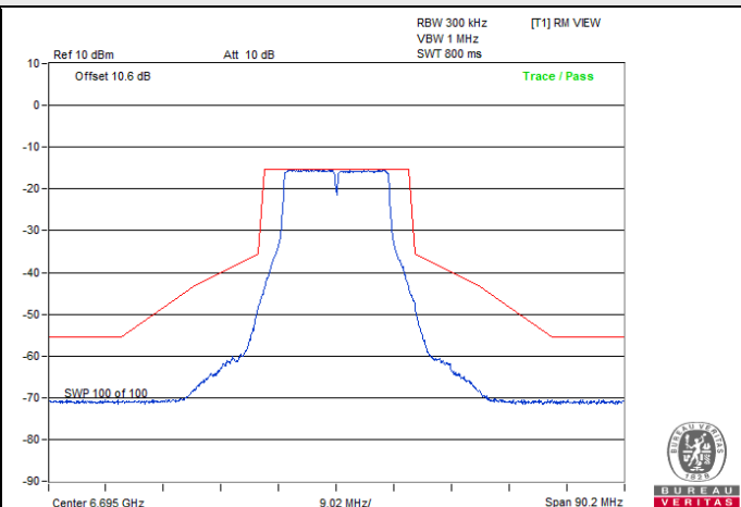
802.11be (EHT20) / Chain 3 : CH 149
