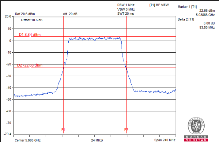
802.11be (EHT80) / Chain 2 : CH 7
