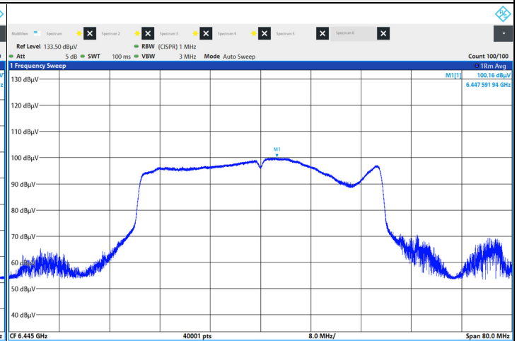
802.11be (EHT40) Beamforming : CH 99
