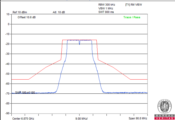
802.11be (EHT20) / Chain 3 : CH 185
