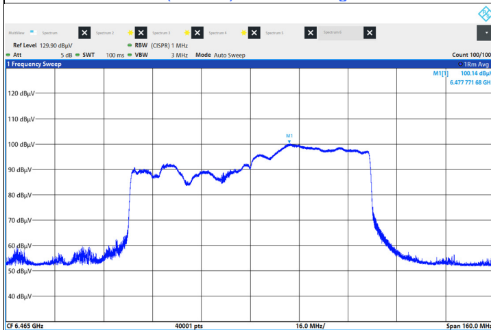
802.11be (EHT80) Beamforming : CH 103
