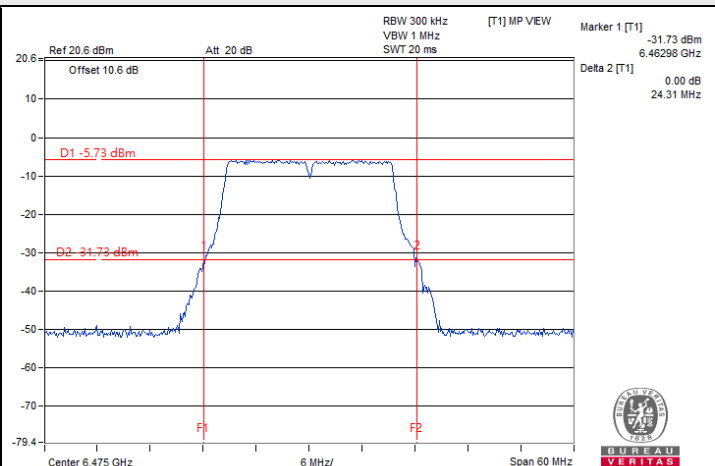
802.11be (EHT20) / Chain 2 : CH 105
