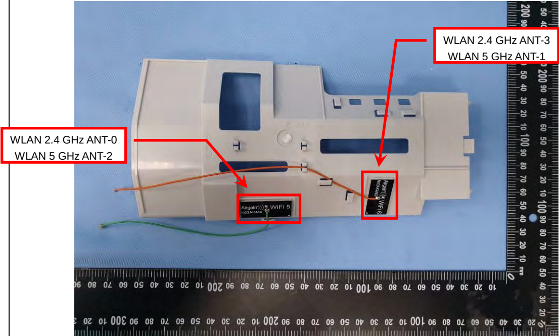
EUT Photo (4)
