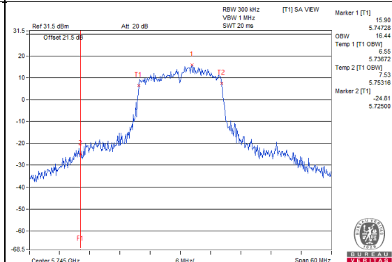
802.11a_Chain3 / CH149
