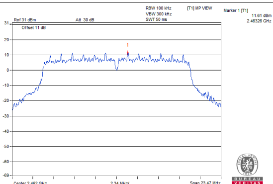
Chain 1 : CH 11
