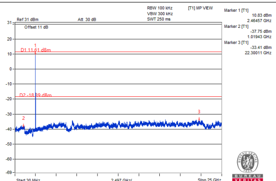
Chain 1 : CH 11
