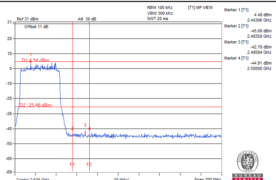
Chain 1 : CH 9 Band edge
