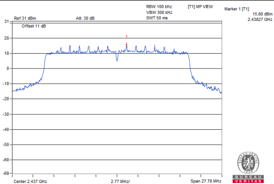
Chain 1 : CH 6
