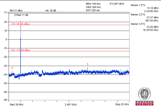
Chain 1 : CH 6
