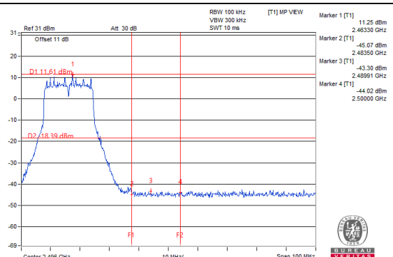
Chain 1 : CH 11 Band edge
