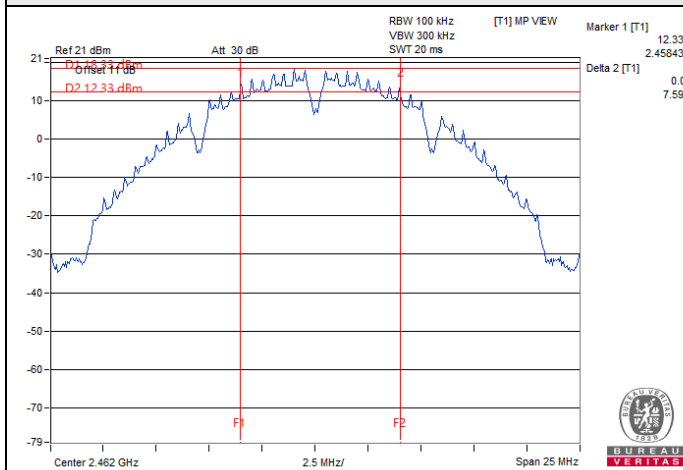
802.11b / Chain 0 : CH 11
