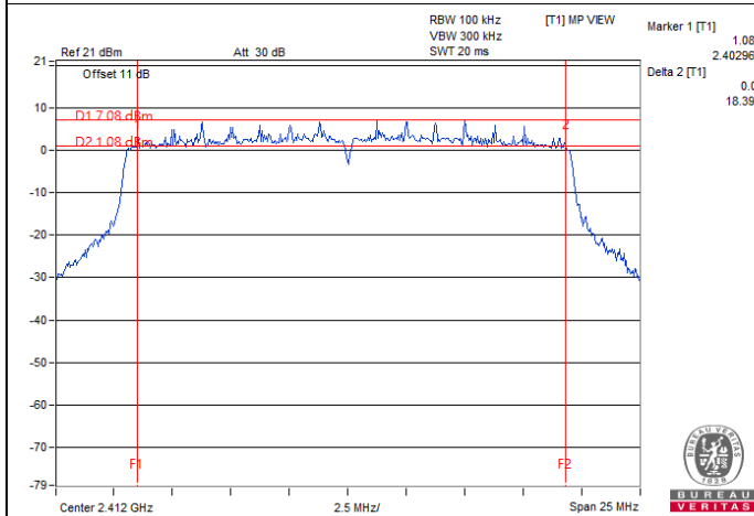
802.11ax (HE20) / Chain 1 : CH 1
