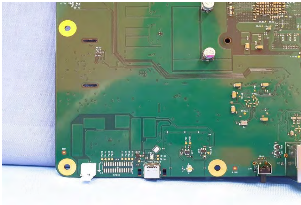
EUT Photo (36)
