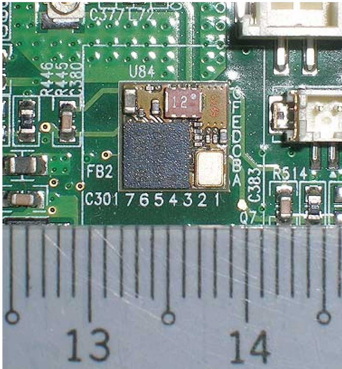
Bluetooth Module
