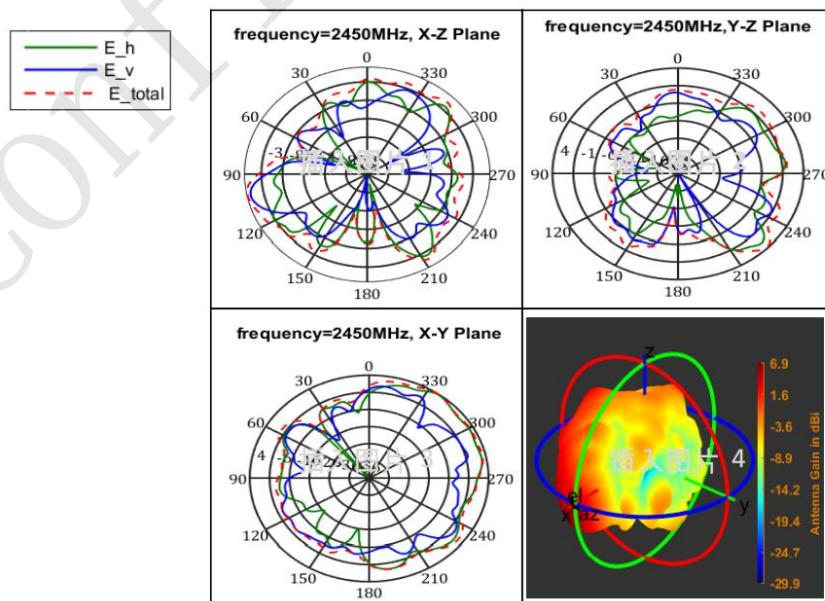
天线辐射方向图 Antenna Radiation Pattern
