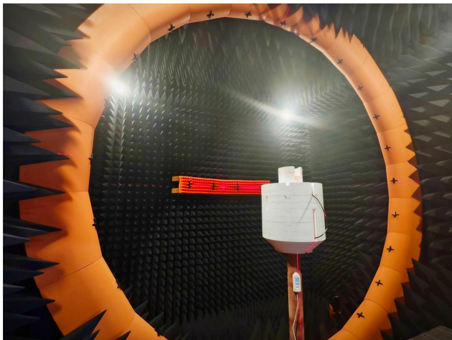
探头微波暗室
