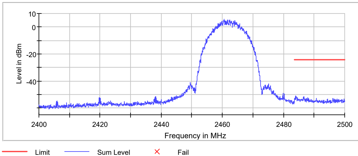
Band Edge
