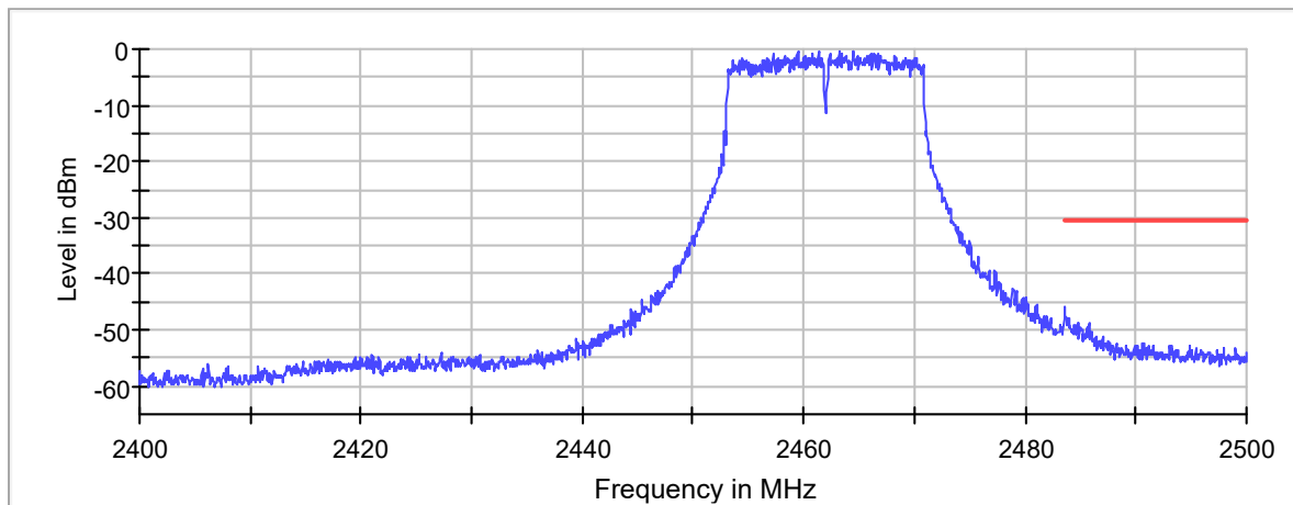
Band Edge
