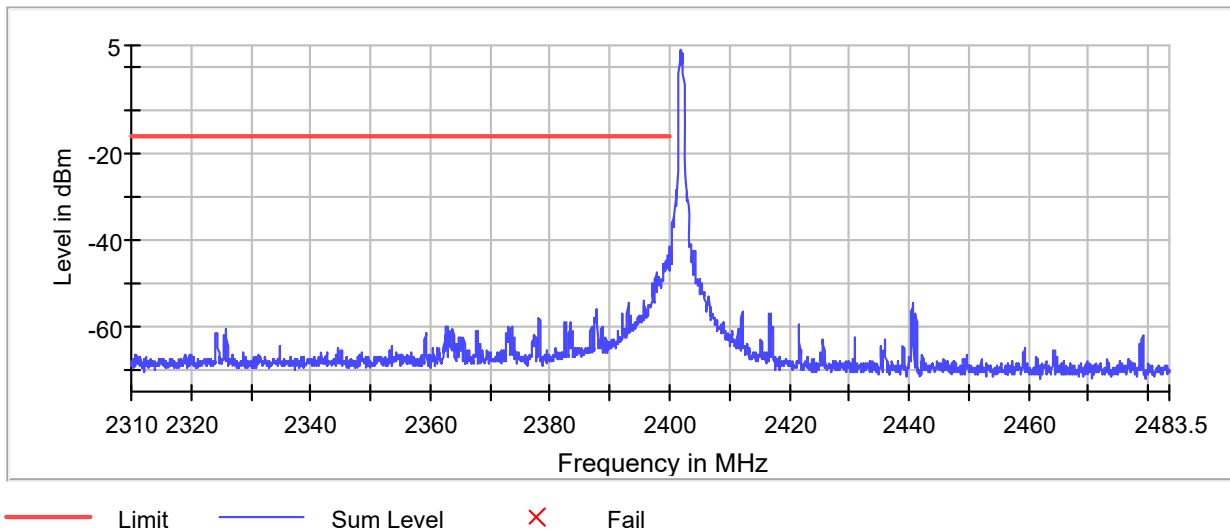
Band Edge
