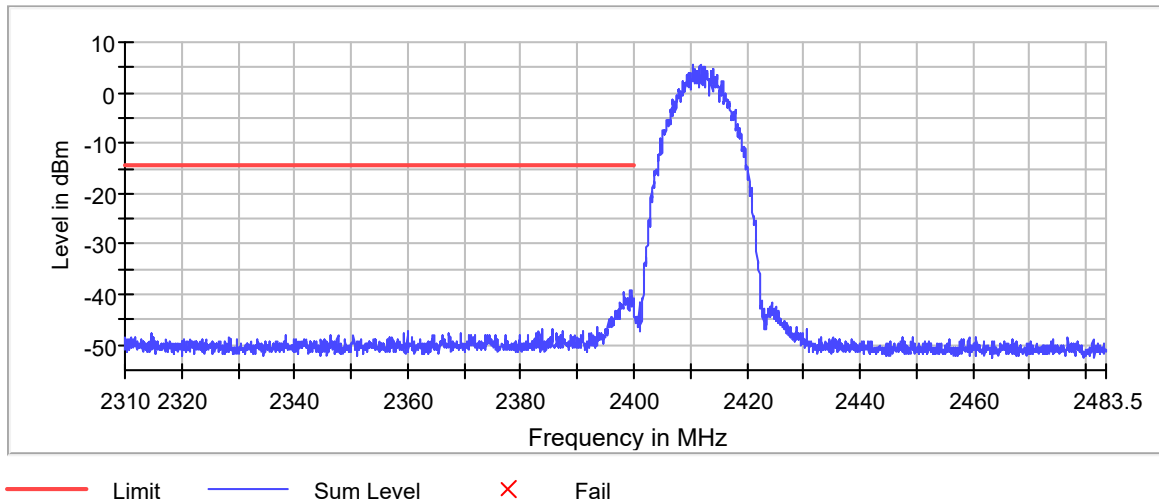
Band Edge
