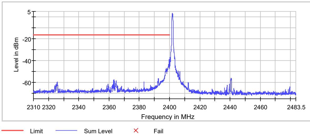
Band Edge
