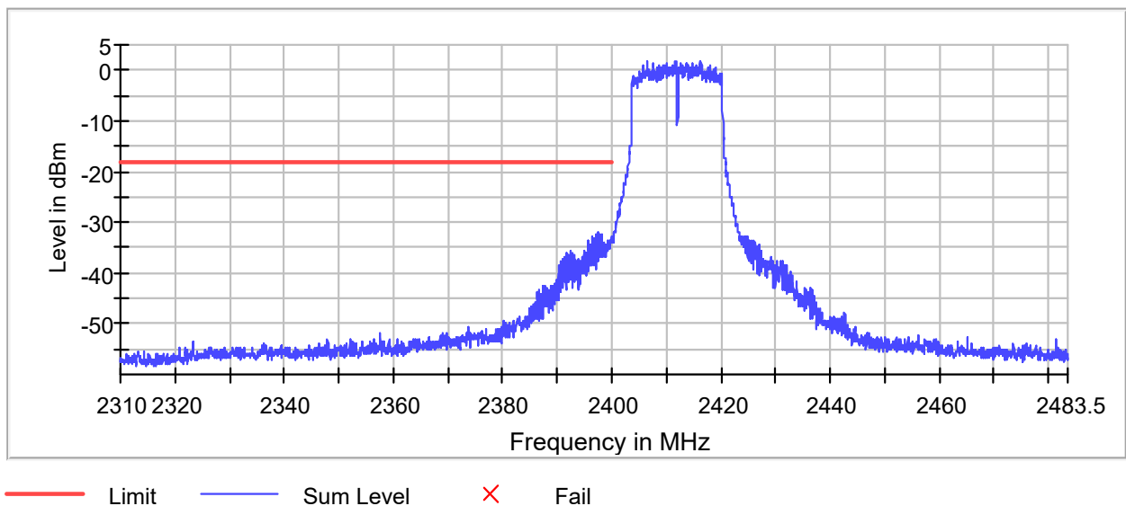
Band Edge
