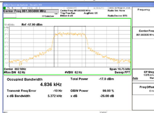
P25 II-CP (Input)
