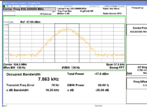
P25 I-P (Input)
