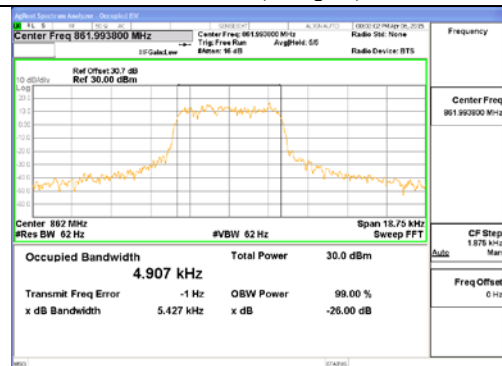
P25 II-CP (Output)
