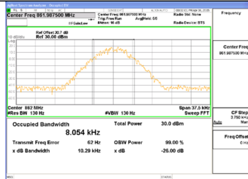
P25 I-P (Output)
