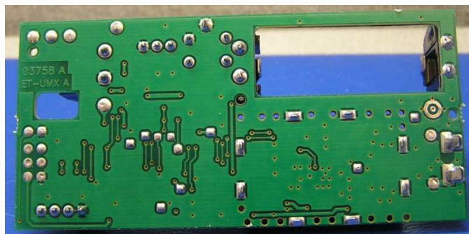
PCB bottomside
