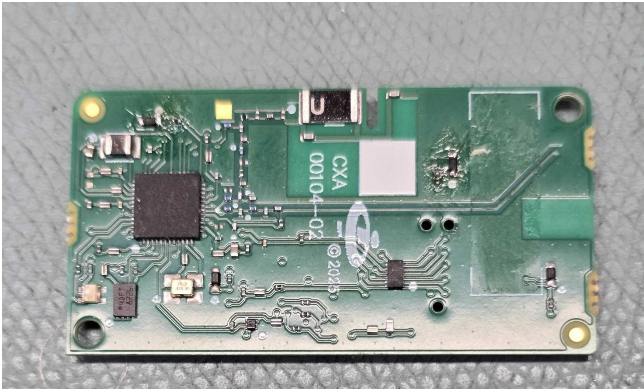
Bottom Main PCA EN2244
