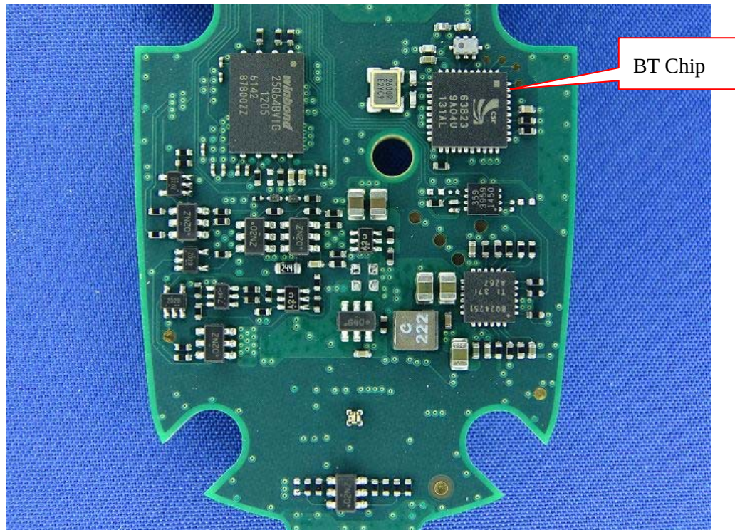
(17) EUT Photo
