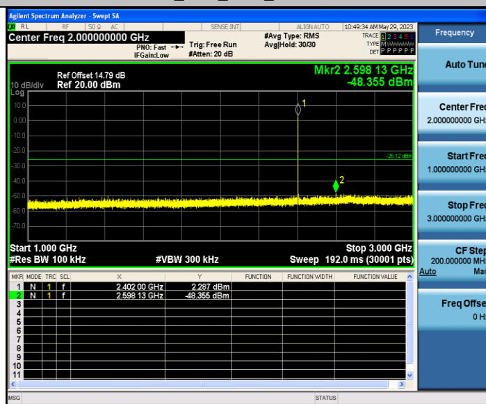
DH5_Ant1_2402_1000~3000
