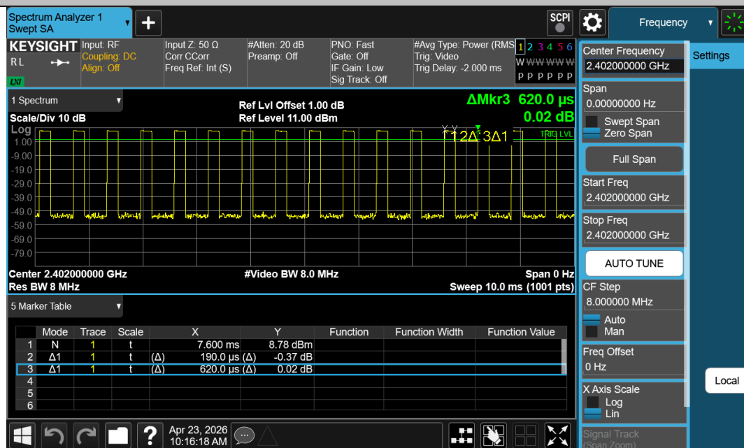
NTNV-BLE_2M-Ant1-2402
