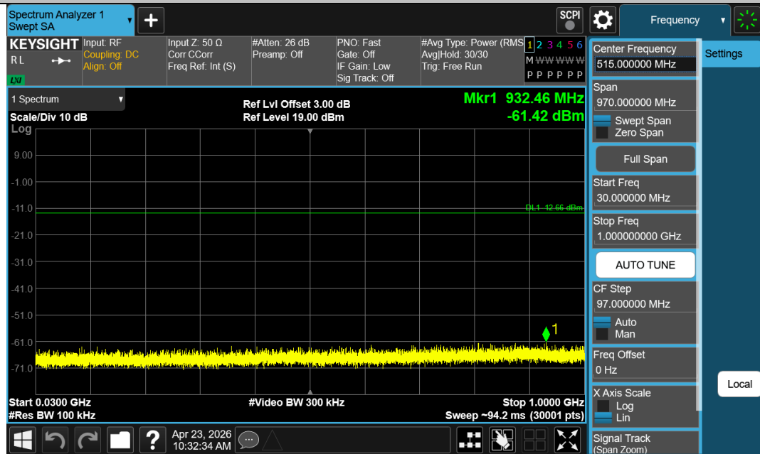
BLE_2M-Ant1-2440-30~1000-PASS
