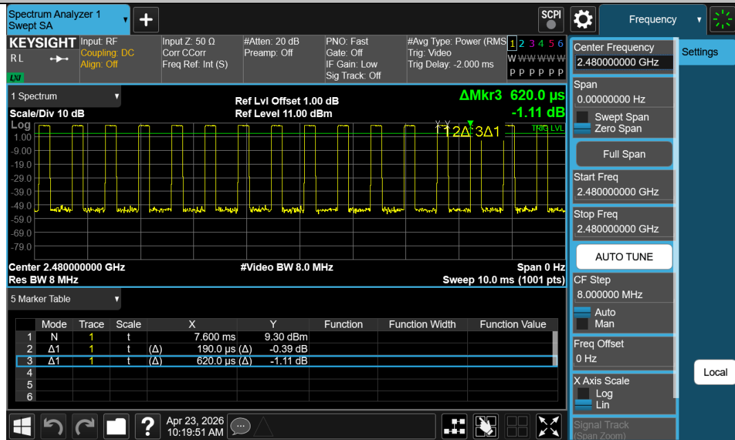
NTNV-BLE_2M-Ant1-2480
