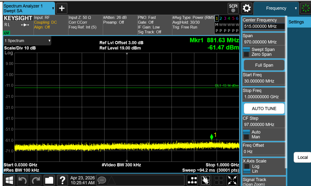
BLE_2M-Ant1-2402-30~1000-PASS
