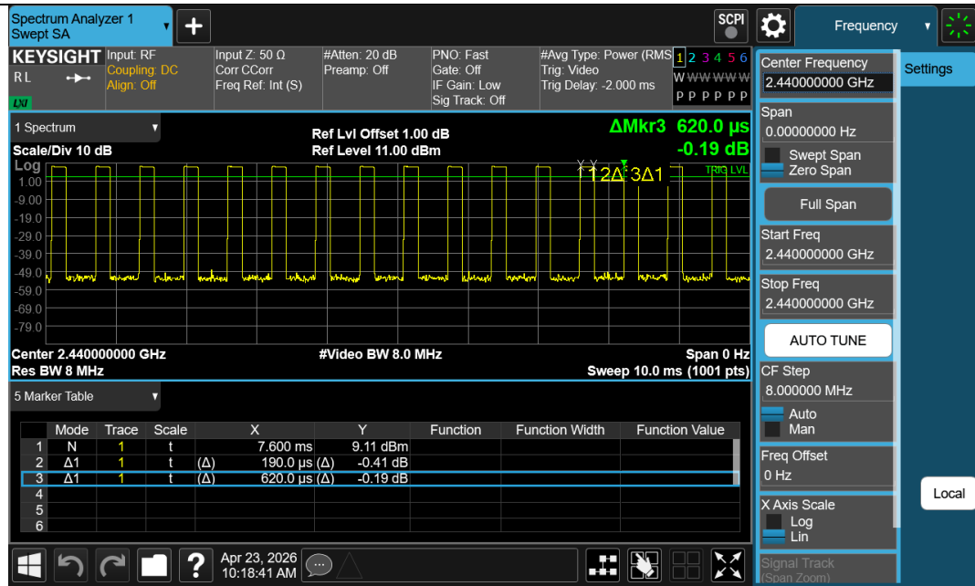
NTNV-BLE_2M-Ant1-2440
