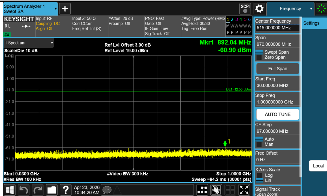
BLE_2M-Ant1-2480-30~1000-PASS
