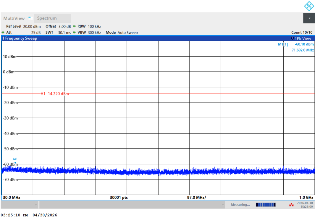
11G-Ant1-2462-30~1000-PASS
