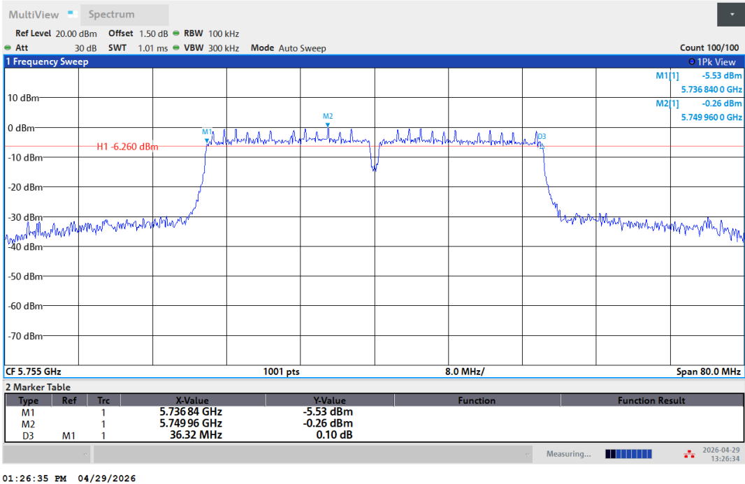
11N40SISO-Ant1-5755-PASS
