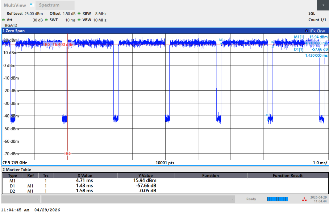
NTNV-11A-Ant1-5745
