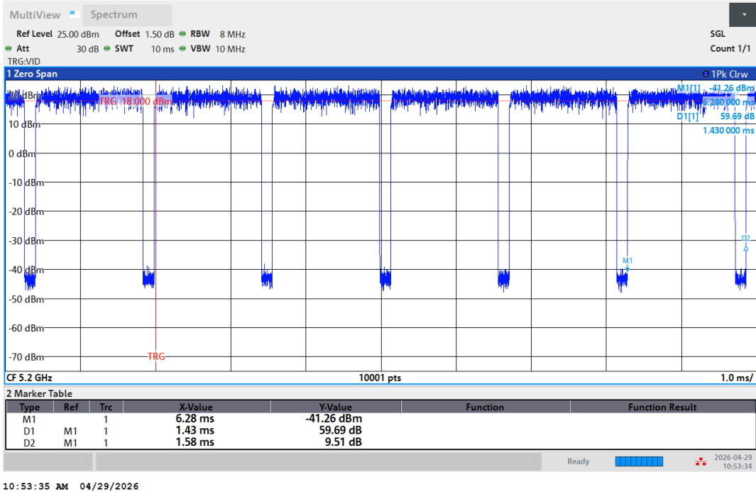
NTNV-11A-Ant1-5200
