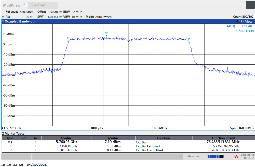
11AC80SISO-Ant1-5775
