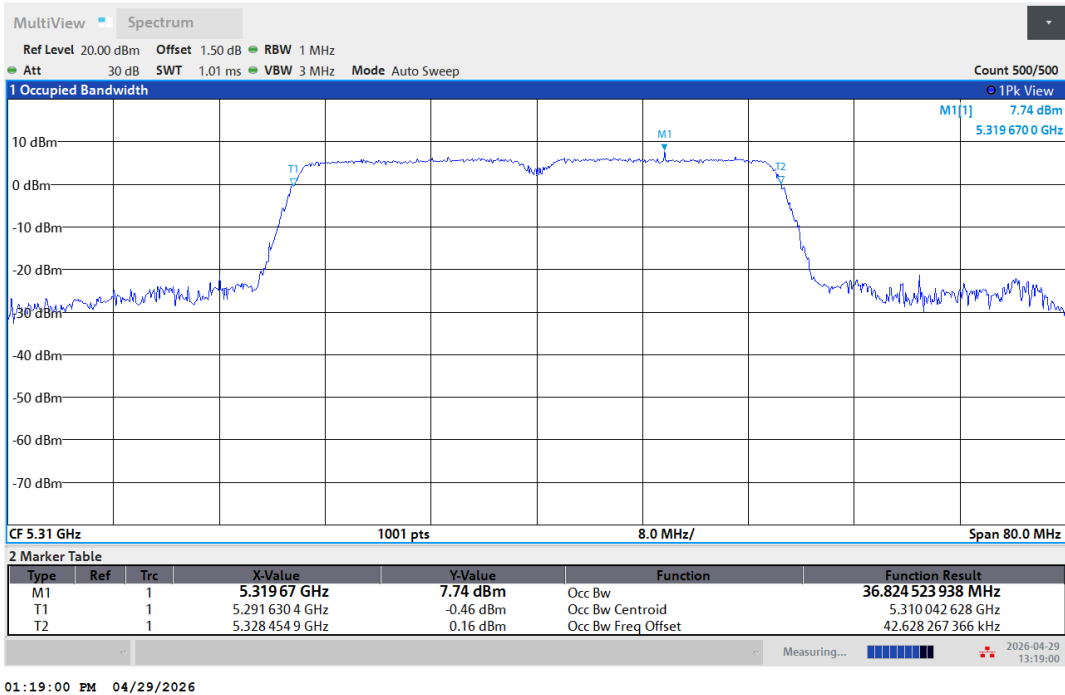
11N40SISO-Ant1-5310
