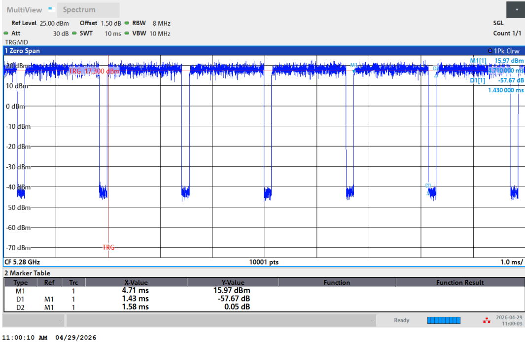
NTNV-11A-Ant1-5280
