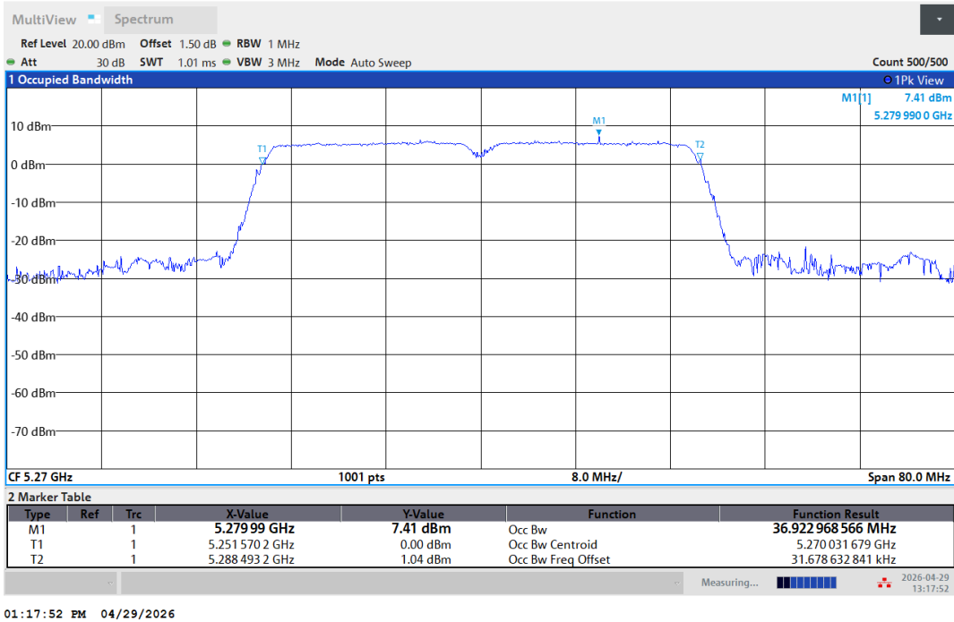
11N40SISO-Ant1-5270
