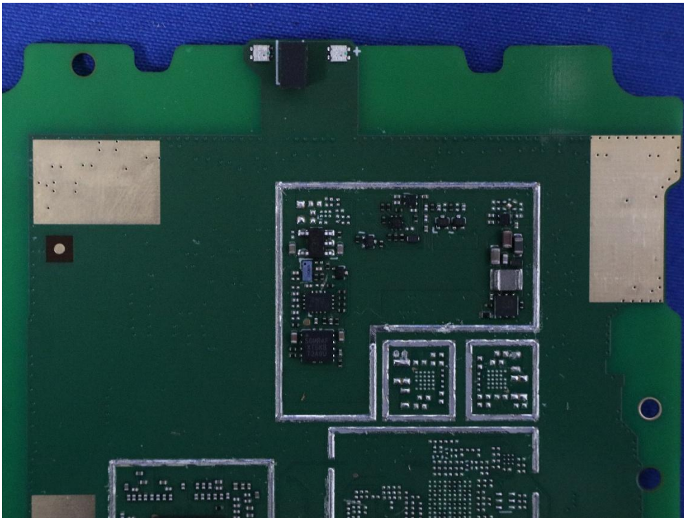
(30) EUT Photo
