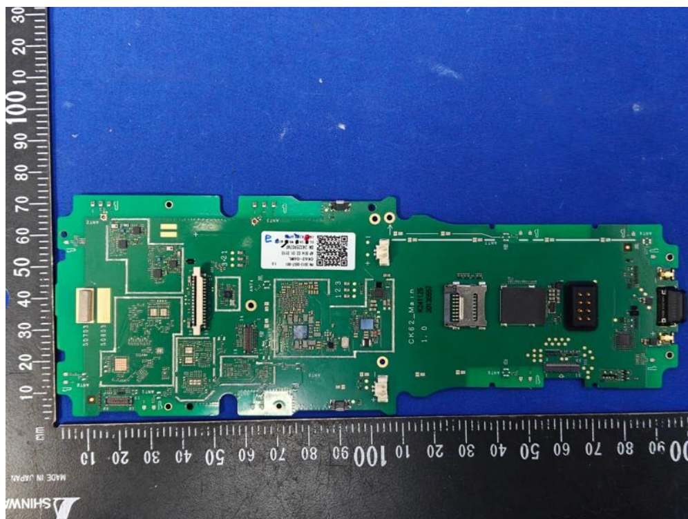
(30) EUT Photo
