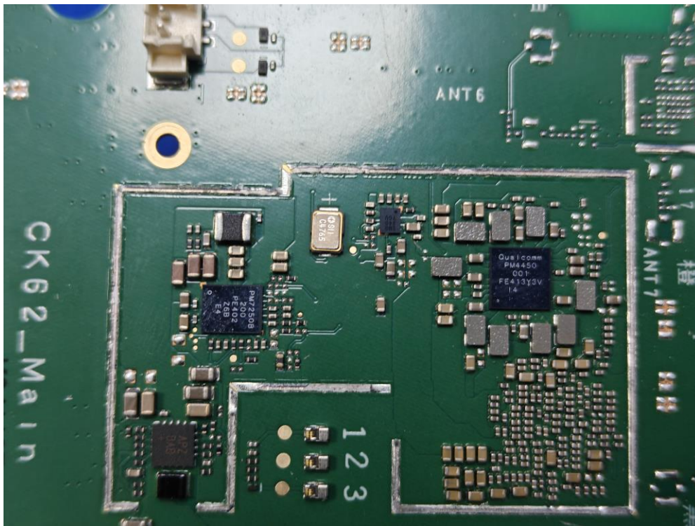
(21) EUT Photo
