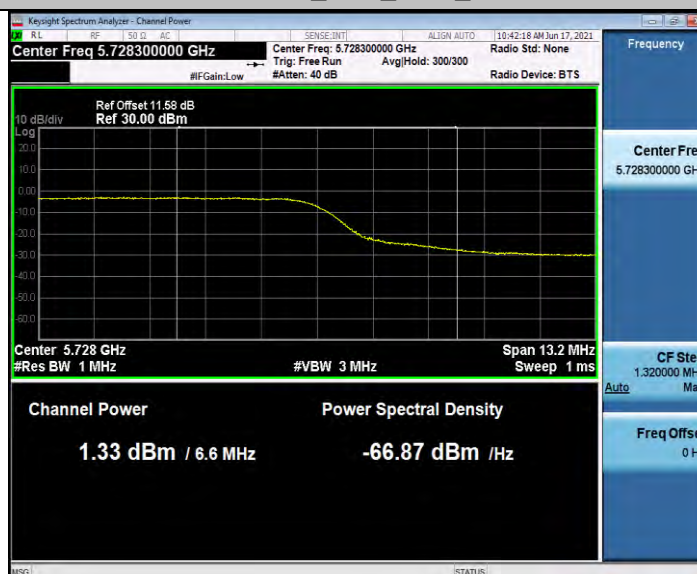
11AC80SISO_Ant1_5690_UNII-2C
