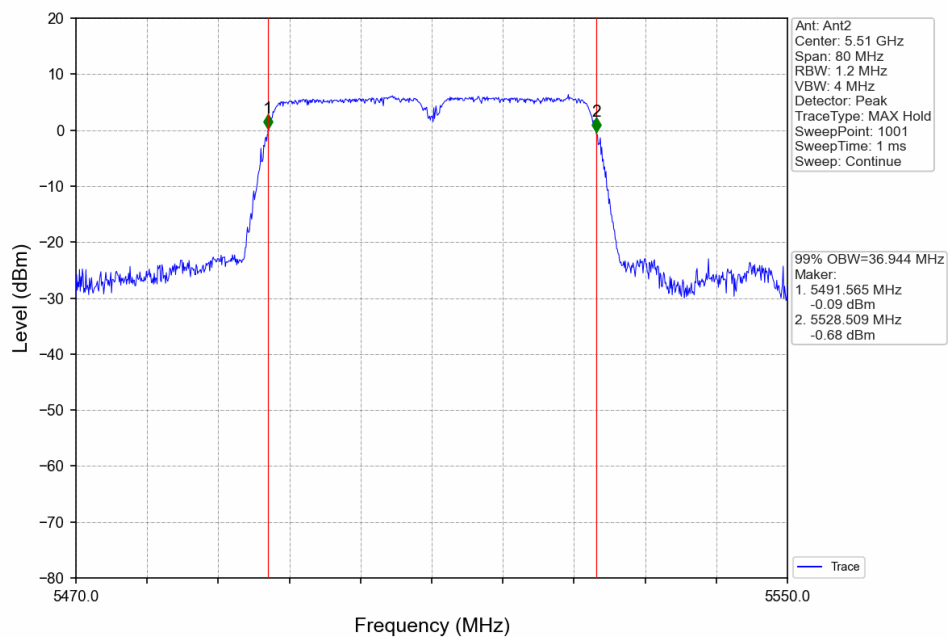
802.11n(HT40)_LCH_5510MHz_Ant2_NTNV
