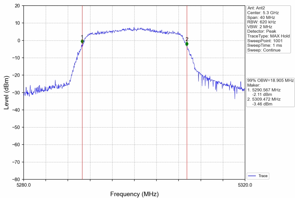
802.11n(HT20)_MCH_5300MHz_Ant2_NTNV
