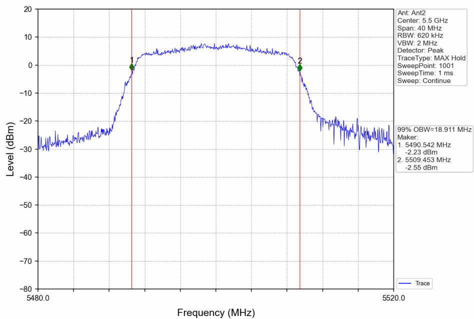
802.11n(HT20)_LCH_5500MHz_Ant2_NTNV
