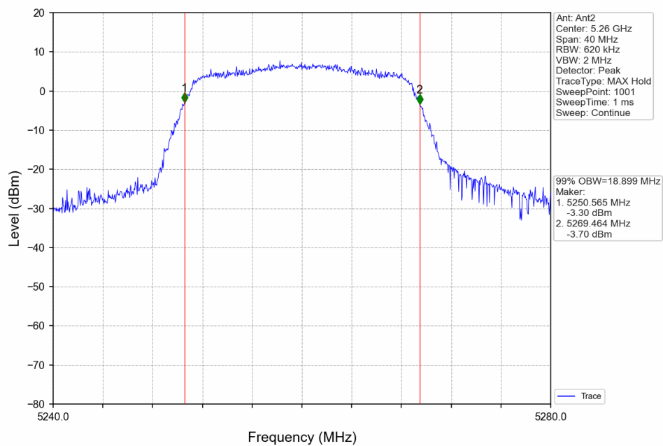
802.11n(HT20)_LCH_5260MHz_Ant2_NTNV
