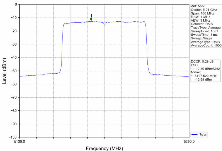
802.11ax(HEW80)_MCH_5210MHz_Ant2_NTNV
