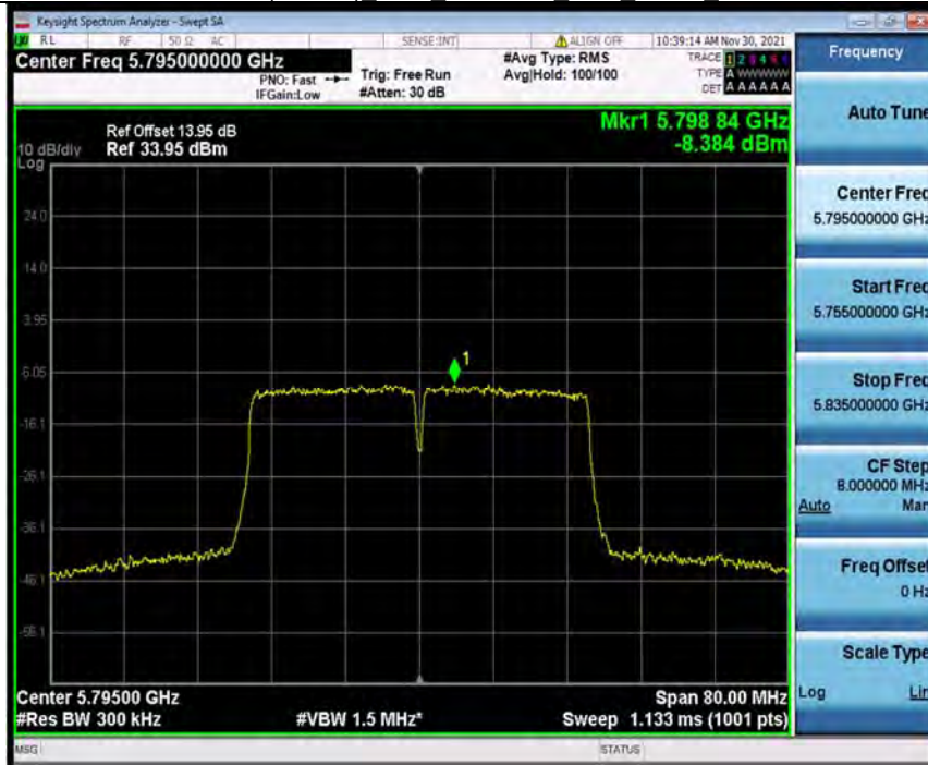
802.11ac(VHT40) HCH 5795MHz Ant2 NTNv MIMO
