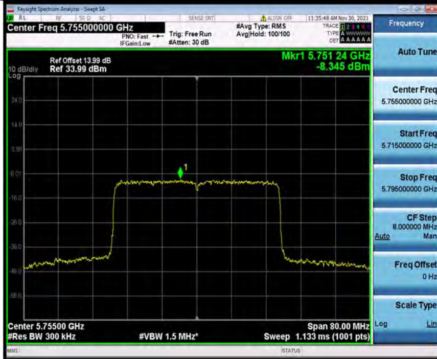
802.11ax(HEW40) LCH_5755MHz Ant2 NTNv MIMO
