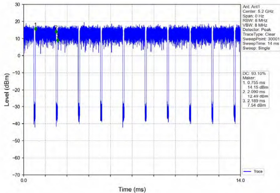
802.11n(HT20) MCH_5200MHz_Ant1_NTNV
