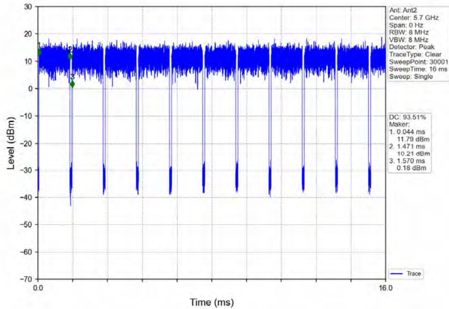
802.11a_LCH_5745MHz_Ant2_NTNV
