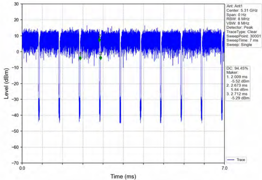
802.11n(HT40) HCH_5310MHz_Ant1_NTNV
