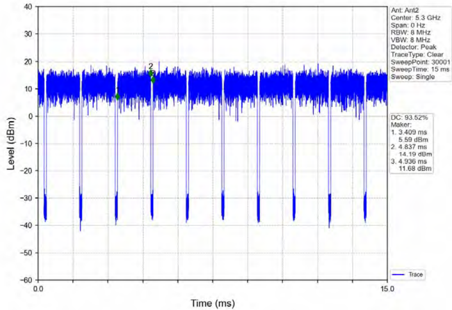
802.11a_HCH_5320MHz_Ant2_NTNV
