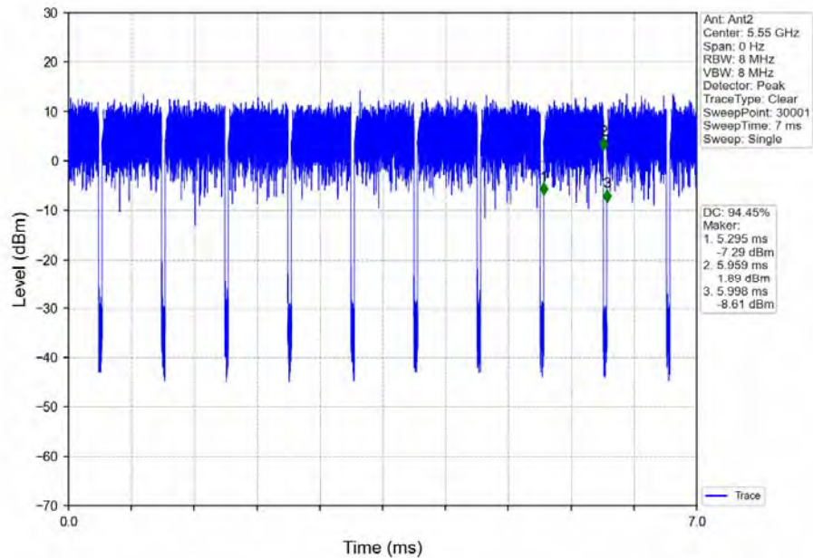
802.11n(HT40) MCH_5550MHz_Ant2_NTNV
