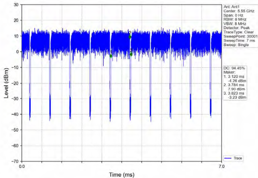
802.11n(HT40) MCH_5550MHz_Ant1_NTNV
