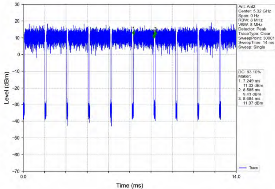
802.11n(HT20)_HCH_5320MHz_Ant2_NTNV
