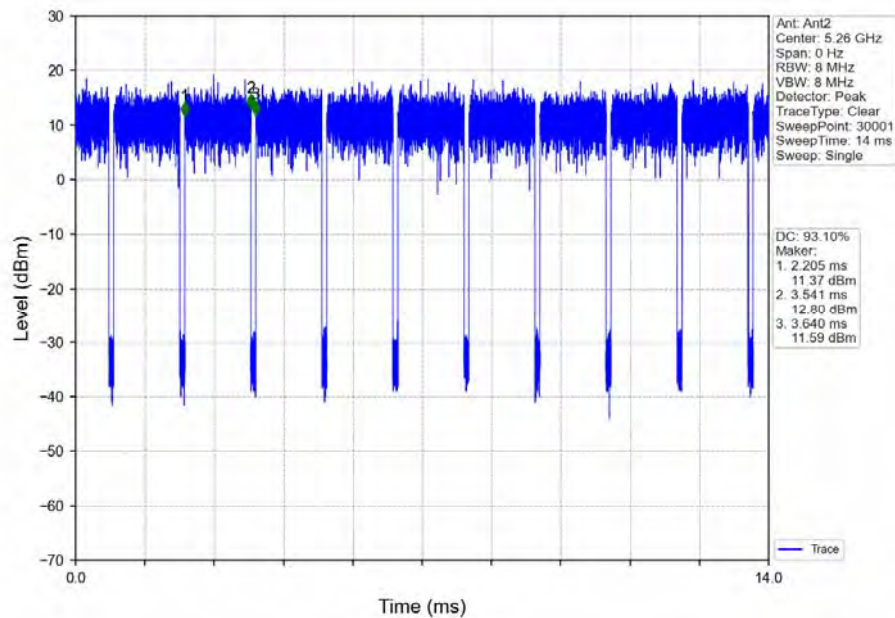
802.11n(HT20)_LCH_5260MHz_Ant2_NTNV
