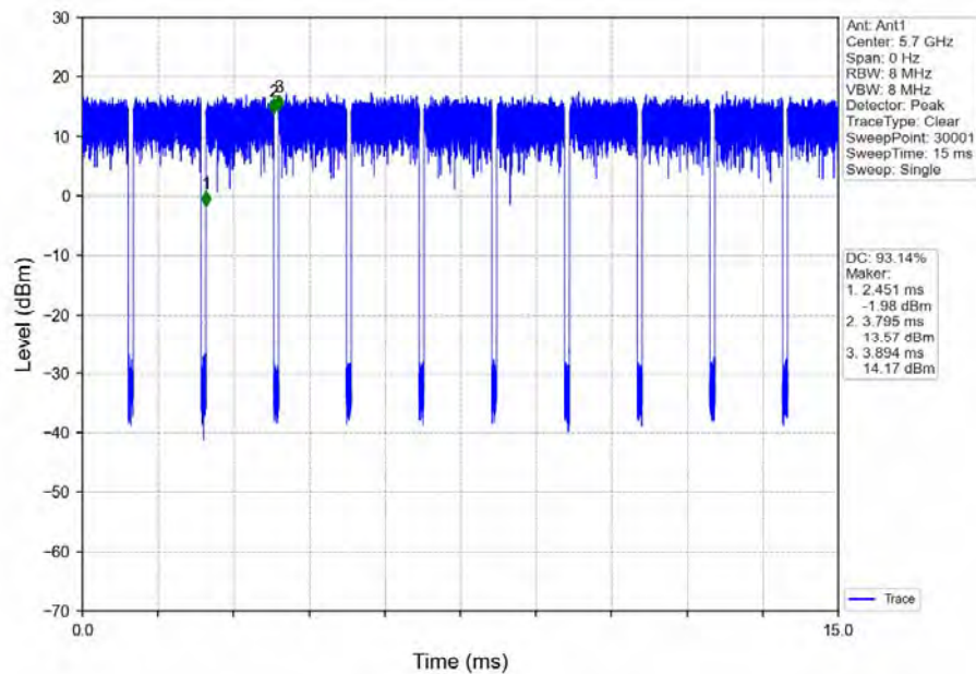
802.11ac(VHT20) HCH_5700MHz_Ant1_NTNV
