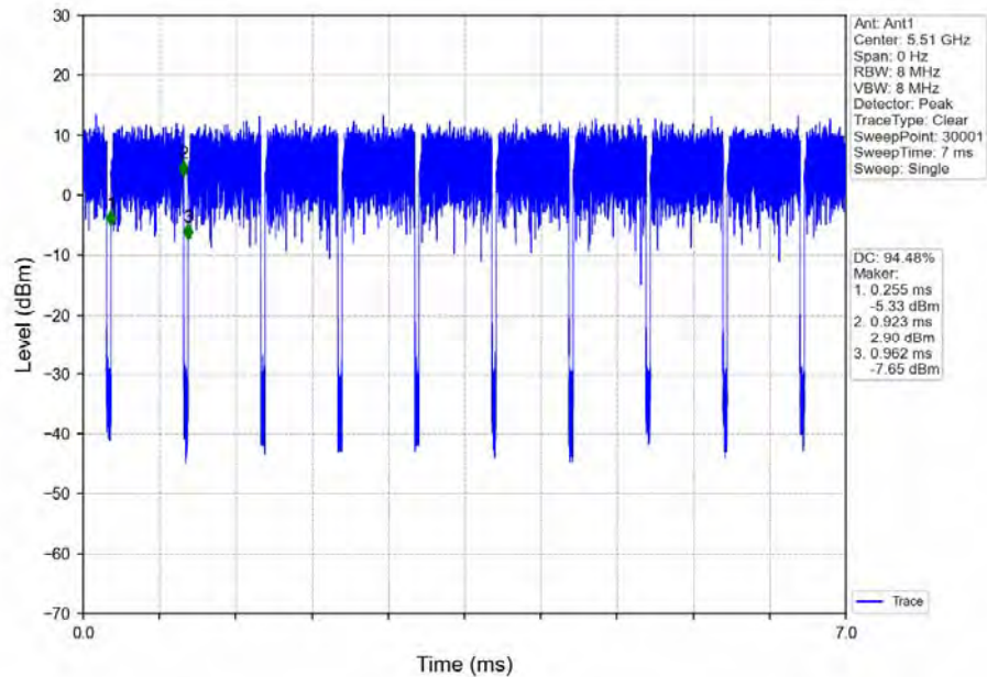
802.11ac(VHT40) LCH_5510MHz_Ant1_NTNV
