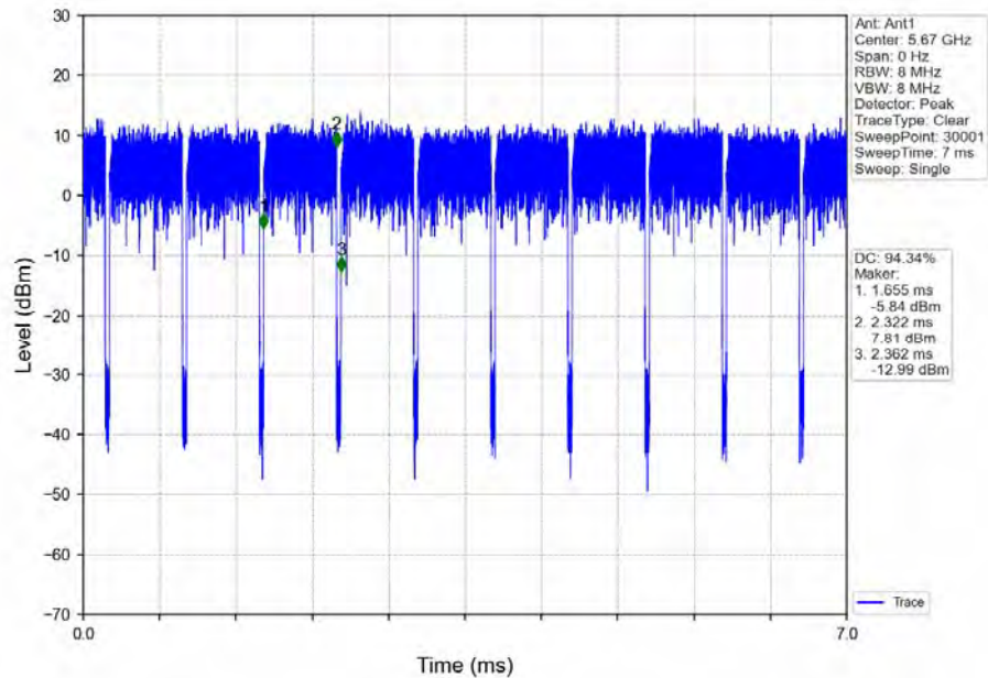
802.11ac(VHT40) HCH_5670MHz_Ant1_NTNV
