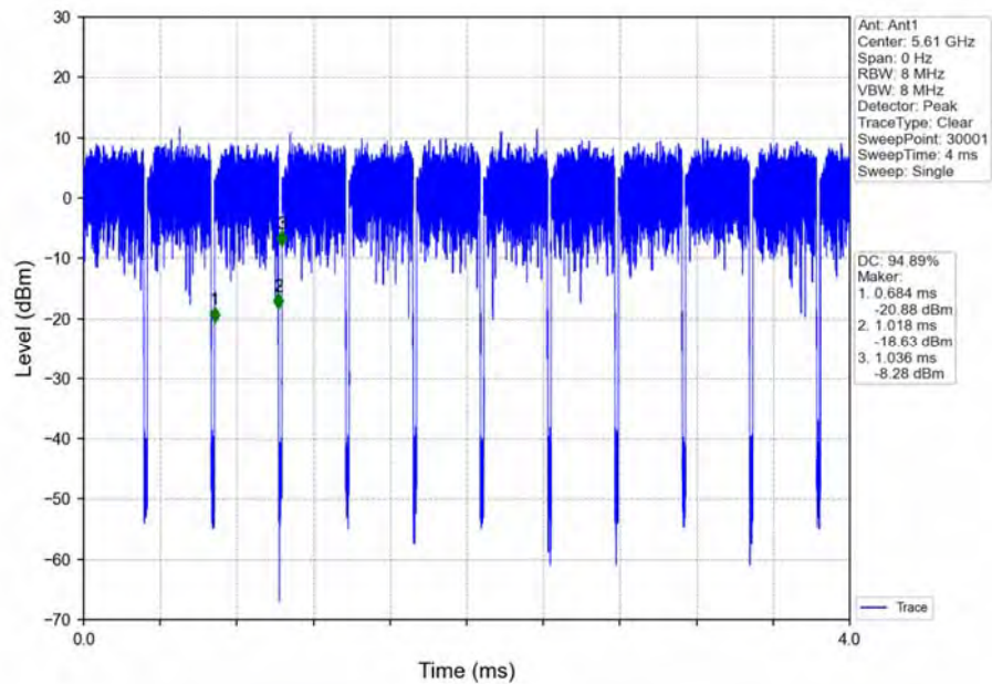
802.11ac(VHT80)_HCH_5610MHz_Ant1_NTNV
