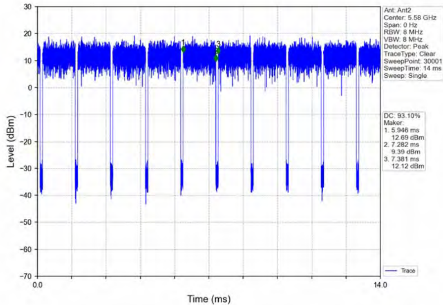
802.11n(HT20) MCH_5580MHz_Ant2_NTNV
