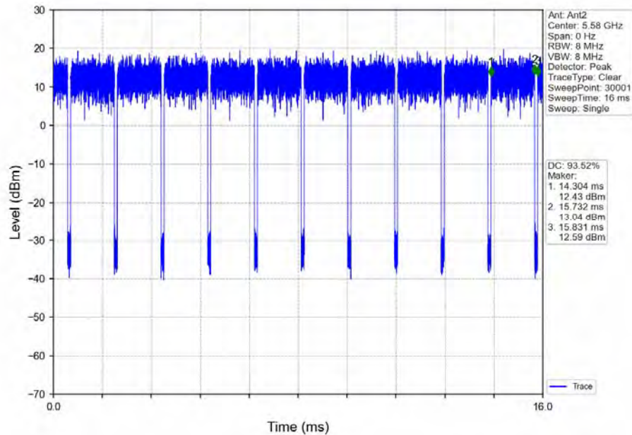
802.11a_MCH_5580MHz_Ant2_NTNV
