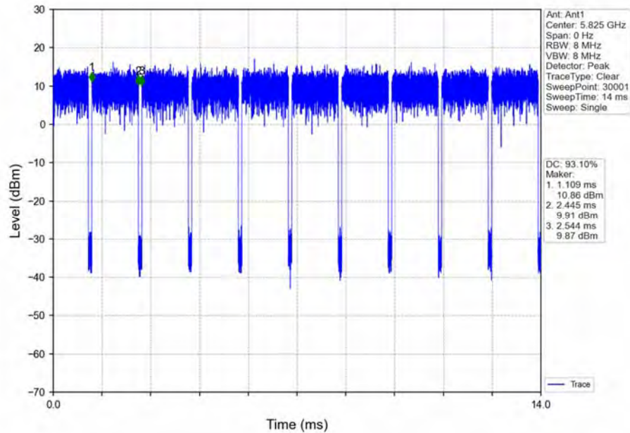
802.11n(HT20)_HCH_5825MHz_Ant1_NTNV
