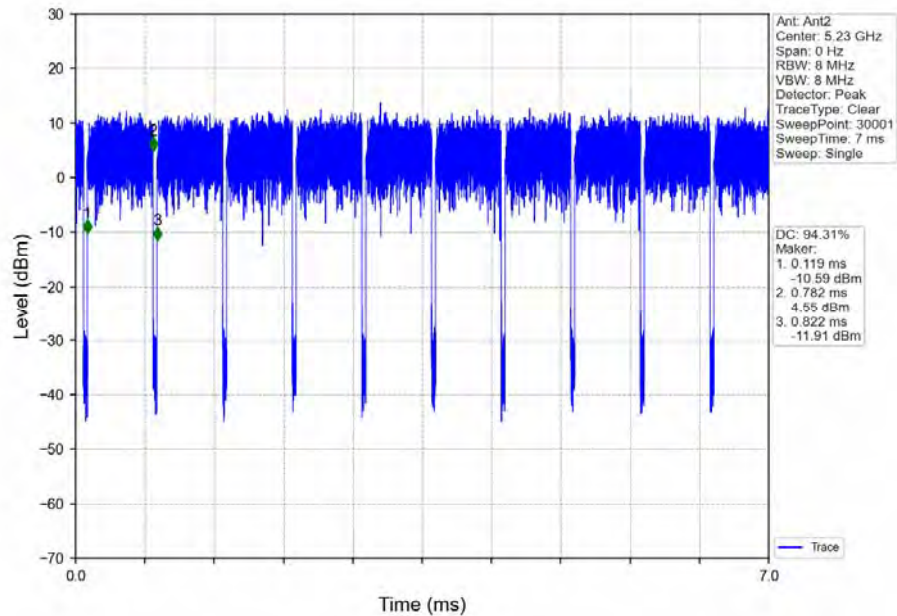
802.11n(HT40) HCH_5230MHz_Ant2_NTNV
