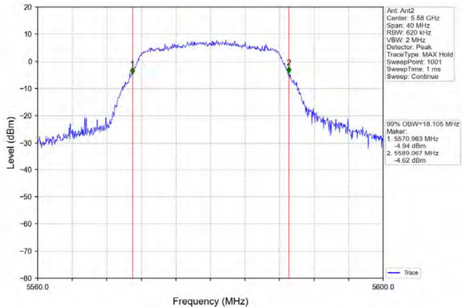
802.11a_MCH_5580MHz_Ant2_NTNV
