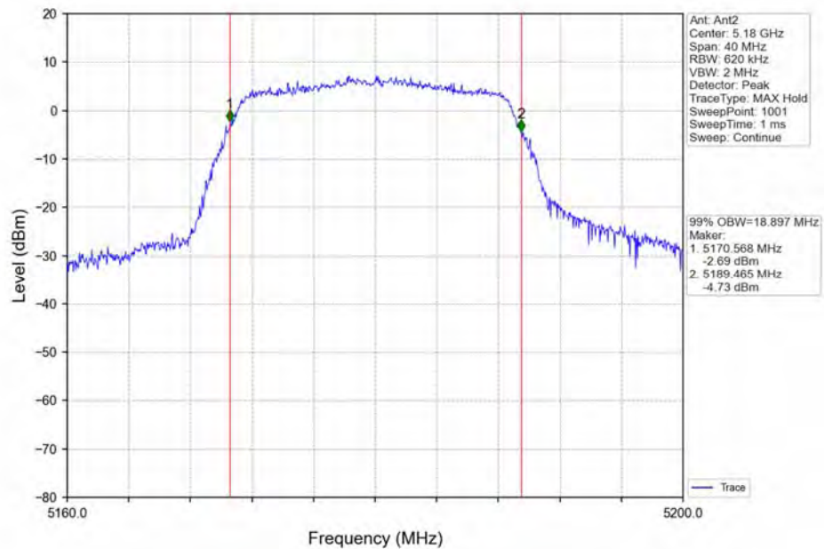
802.11n(HT20) LCH_5180MHz_Ant2_NTNV
