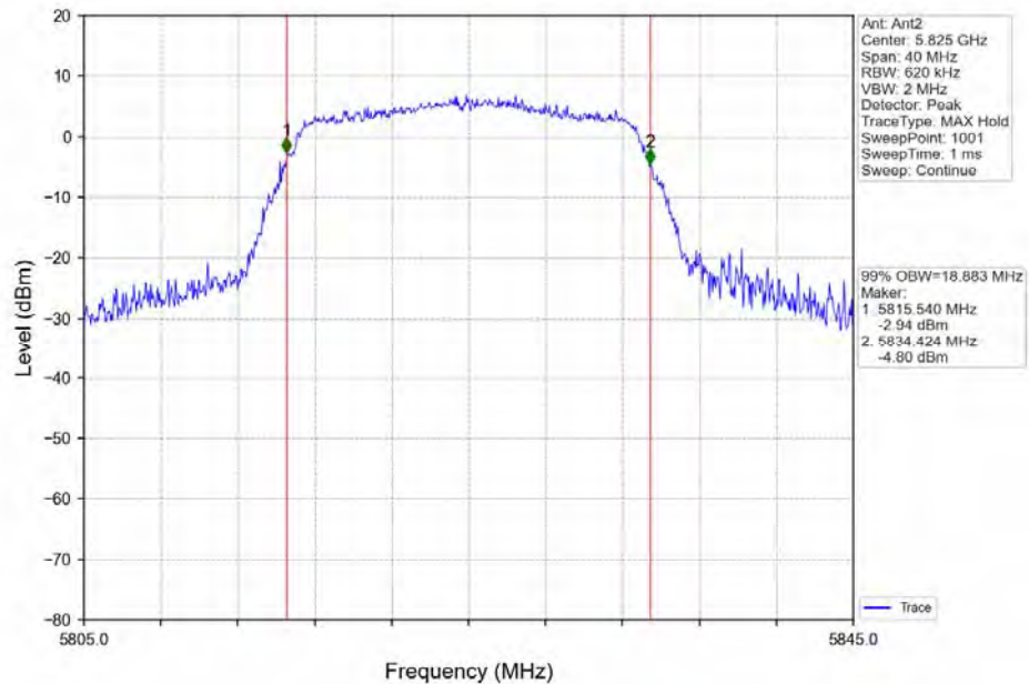
802.11n(HT20)_HCH_5825MHz_Ant2_NTNV
