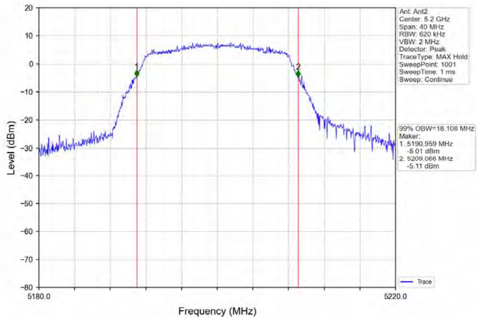
802.11a_MCH_5200MHz_Ant2_NTNV
