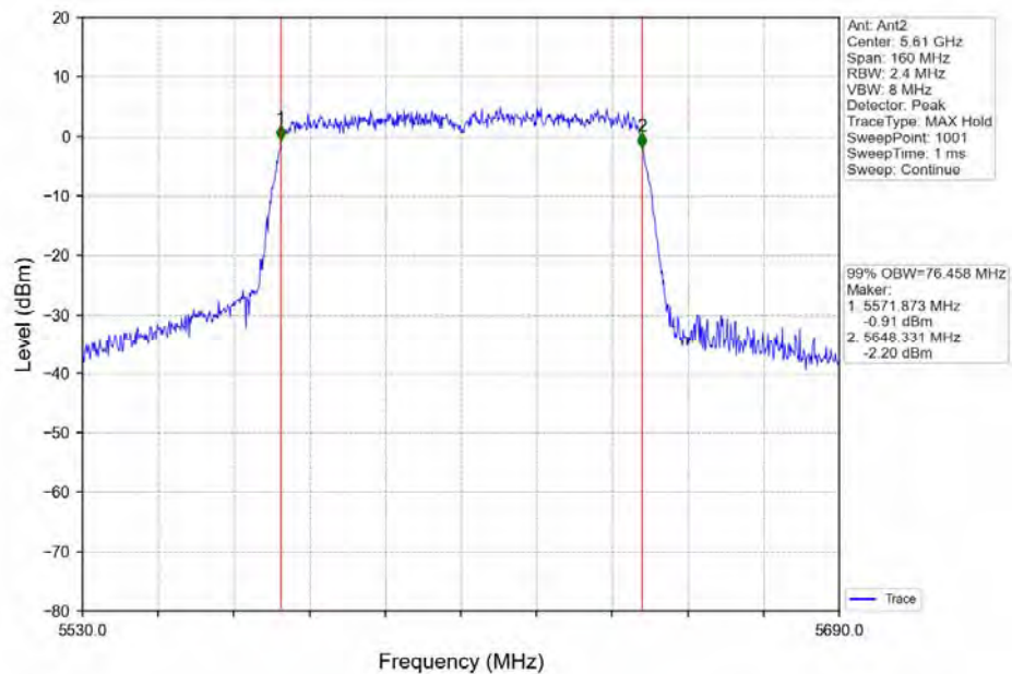
802.11ac(VHT80) HCH_5610MHz_Ant2_NTNV
