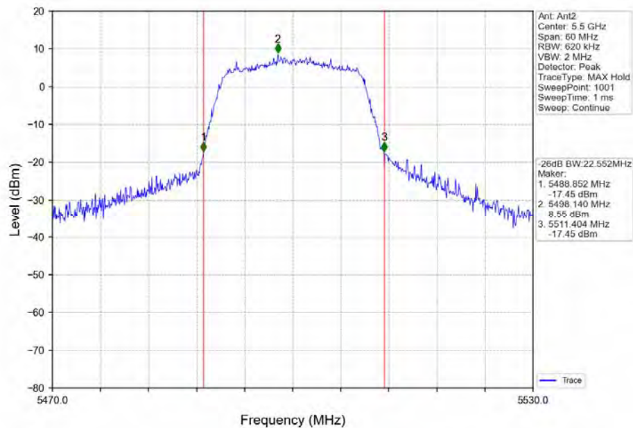
802.11n(HT20) LCH_5500MHz_Ant2_NTNV
