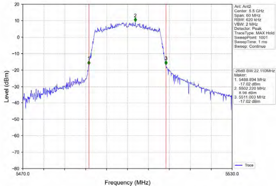
802.11ax(HEW20)_LCH_5500MHz_Ant2_NTNV
