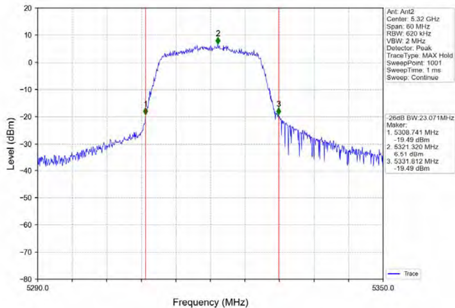
802.11ac(VHT20) HCH_5320MHz_Ant2_NTNV
