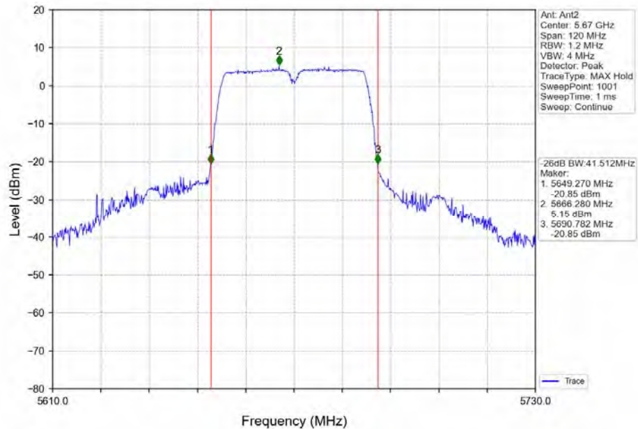
802.11ac(VHT40) HCH_5670MHz_Ant2_NTNV
