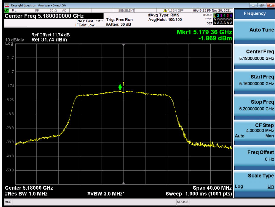
802.11ac(VHT20) LCH 5180MHz Ant2 NTNv MIMO
