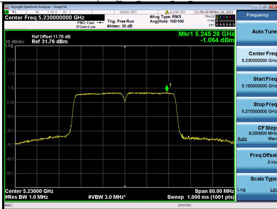
802.11n(HT40) HCH 5230MHz Ant2 NTN
