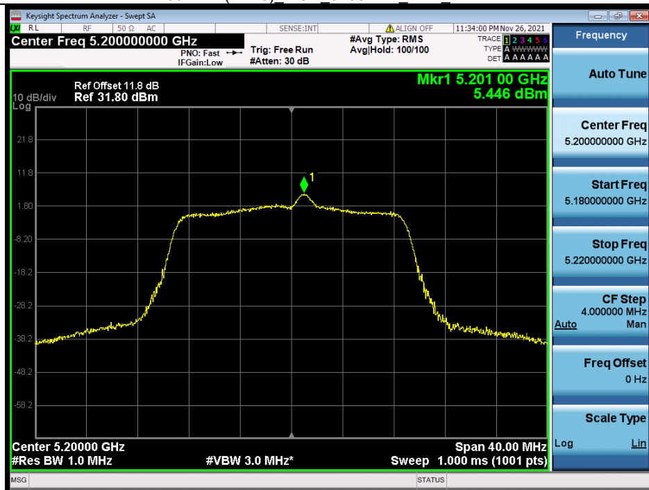
802.11n(HT20) MCH 5200MHz Ant2 NTN
